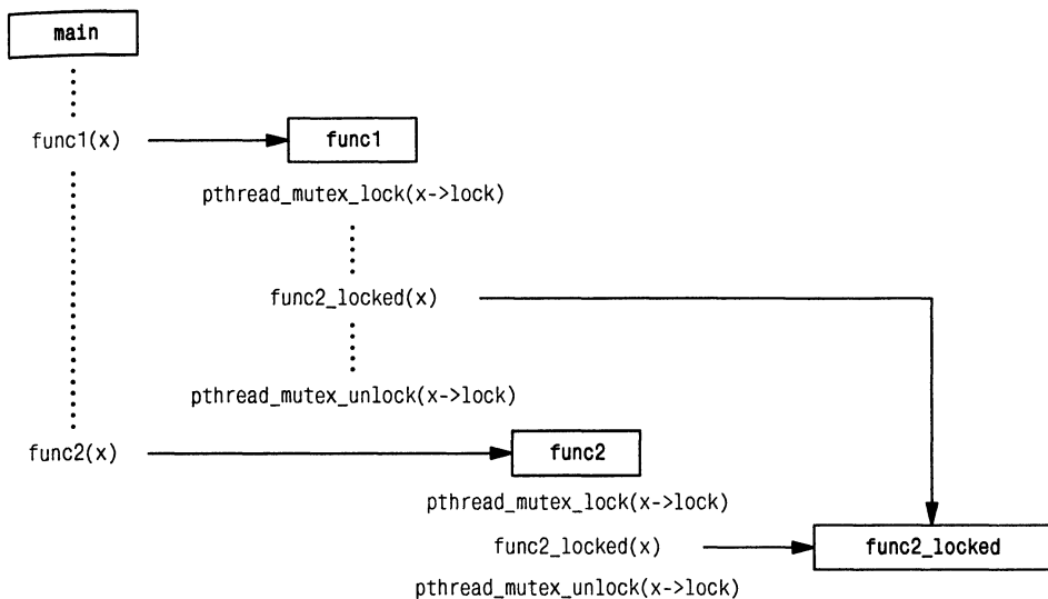
Рис. 12.2. Отказ от использования рекурсивной блокировки
