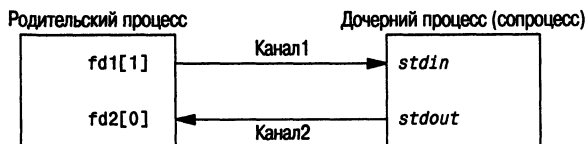
Рис. 15.8. Запись на стандартный ввод и чтение со стандартного вывода сопроцесса
