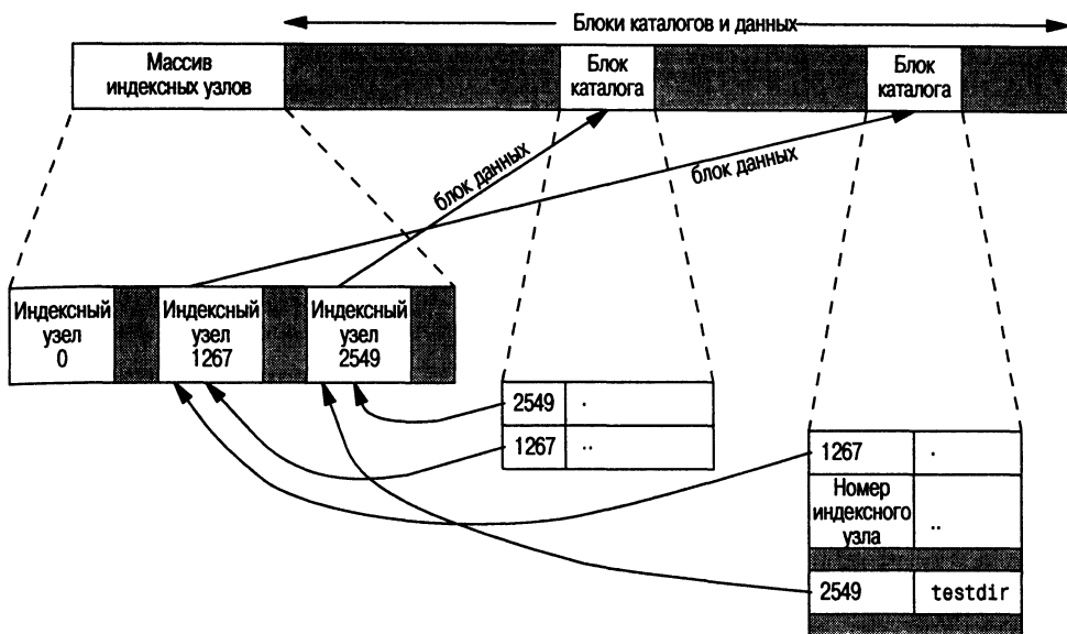
Рис. 4.3. Группа цилиндров после создания каталога testdir
