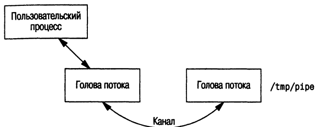
Рис. 17.5. Канал, связанный с именем из файловой системы
