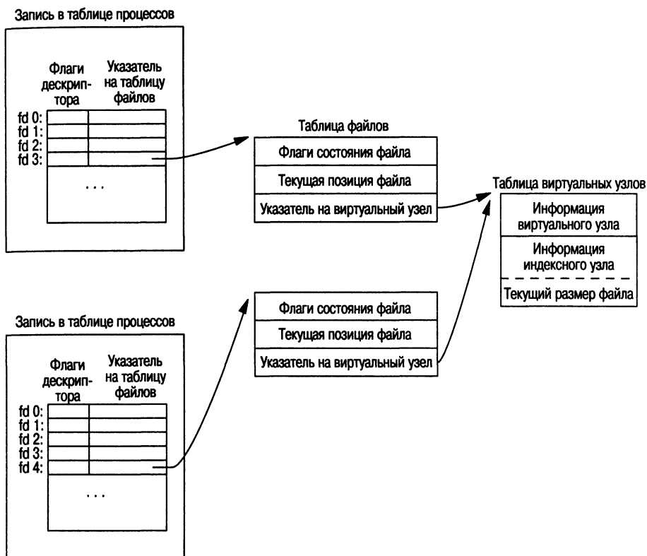
Рис. 3.2. Два независимых процесса открыли один и тот же файл
