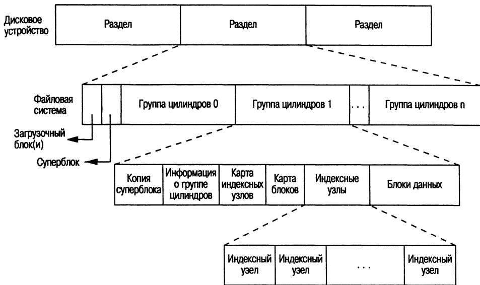
Рис. 4.1. Дисковое устройство, разделы и файловая система
