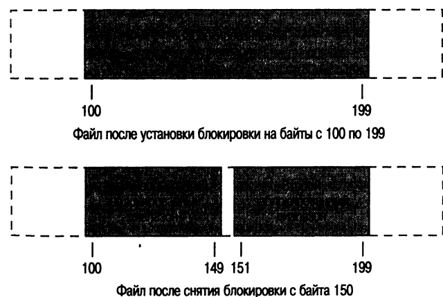
Рис. 14.1. Схема блокировки диапазона байтов
