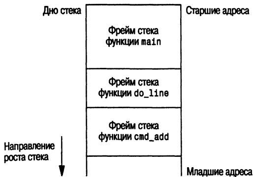
Рис. 7.4. Состояние стека после вызова функции cmd_add
