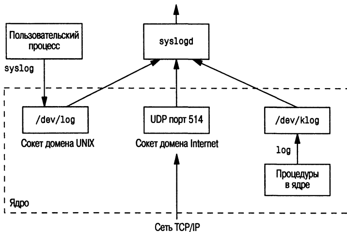
Рис. 13.1. Механизм syslog для BSD-систем
