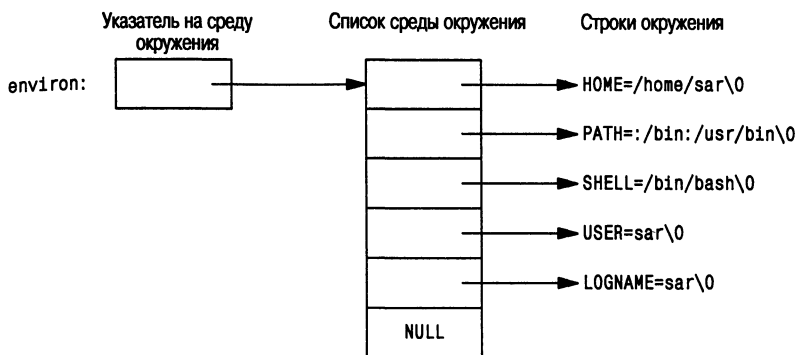
Рис. 7.2. Среда окружения, состоящая из пяти строк
