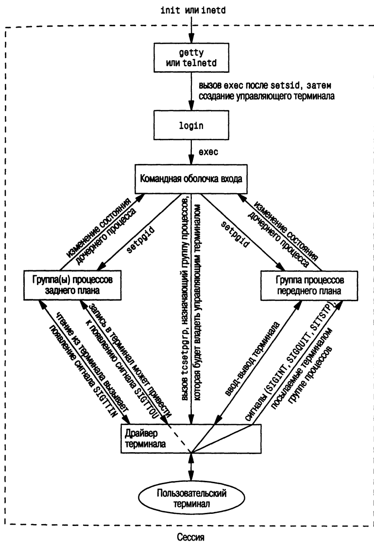
Рис. 9.8. Схема взаимодействия заданий переднего плана и фонового режима с драйвером терминала
