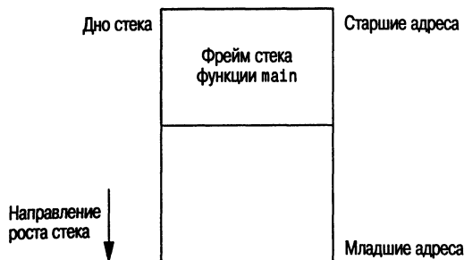
Рис. 7.5. Состояние стека после вызова функции longjmp
