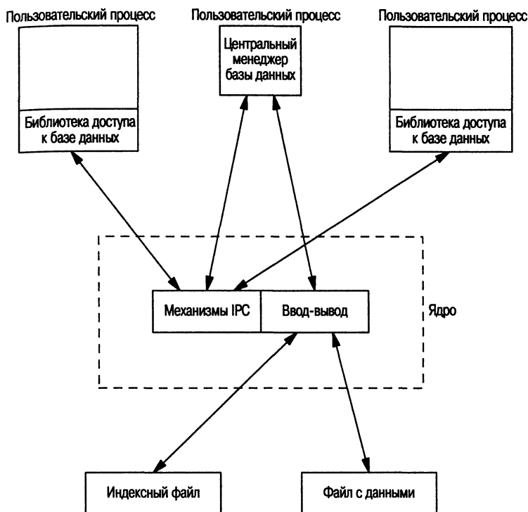
Рис. 20.2. Централизованный доступ к базе данных
