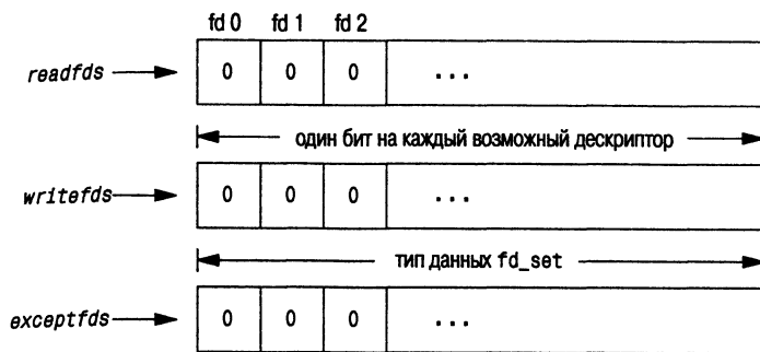
Рис. 14.8. Определение наборов дескрипторов для функции select
