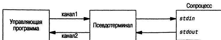
Рис. 19.5. Управление сопроцессом с помощью псевдотерминала
