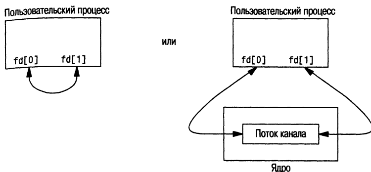
Рис. 17.1. Два взгляда на канал STREAMS
