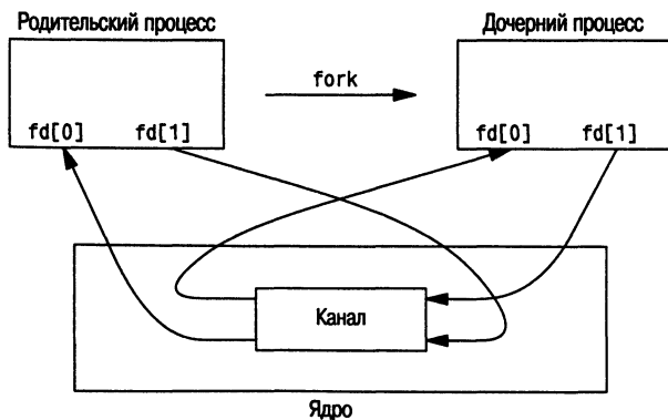
Рис. 15.2. Полудуплексные каналы после вызова функции fork
