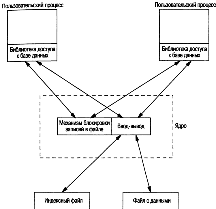
Рис. 20.3. Децентрализованный доступ к базе данных
