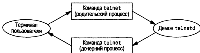
Рис. 14.7. Реализация программы telnet в виде двух процессов
