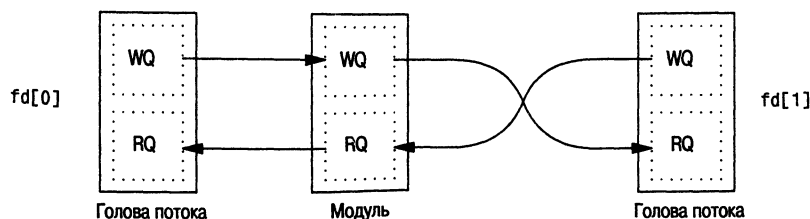
Рис. 17.3. Дополнительный модуль внутри канала STREAMS
