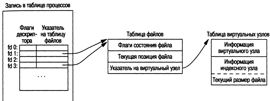
Рис. 3.3. Структуры в ядре после вызова функции dup(1)
