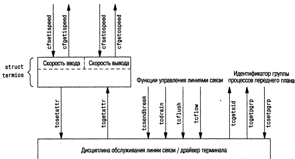
Рис. 18.3. Взаимосвязь функций, предназначенных для работы с терминалами
