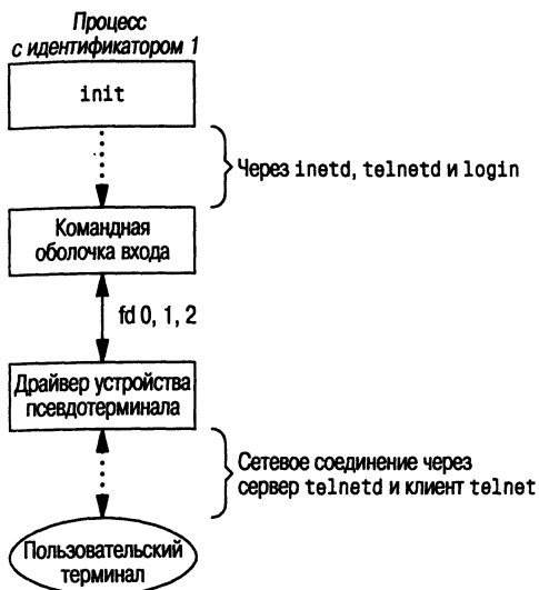
Рис. 9.5. Состояние процессов после входа пользователя через сетевое соединение
