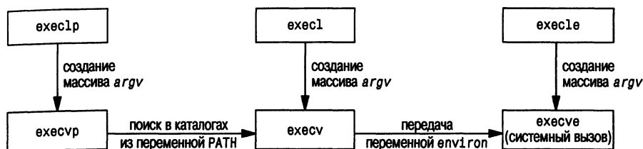
Рис. 8.2. Взаимоотношения между шестью функциями exec
