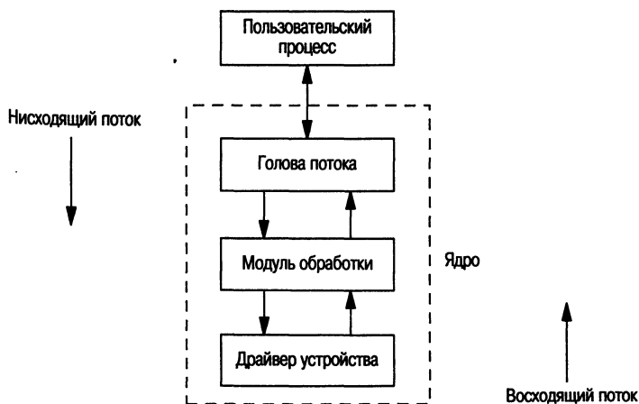
Рис. 14.5. Поток с модулем промежуточной обработки данных
