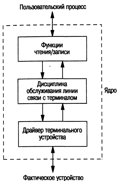
Рис. 18.2. Модуль, реализующий дисциплину обслуживания линии связи с терминалом
