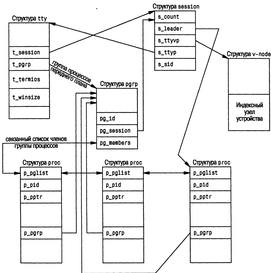
Рис. 9.11. Реализация сессий и групп процессов в ОС FreeBSD
