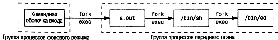
Рис. 10.2. Группы процессов переднего плана и фонового режима
