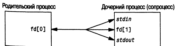
Рис. 17.4. Схема размещения дескрипторов для сопроцесса
