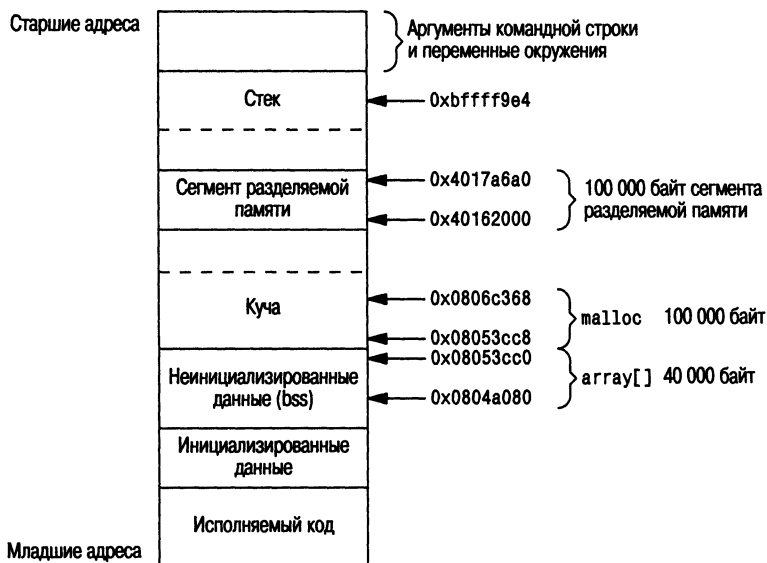
Рис. 15.13. Раскладка памяти в ОС Linux на платформе Intel
