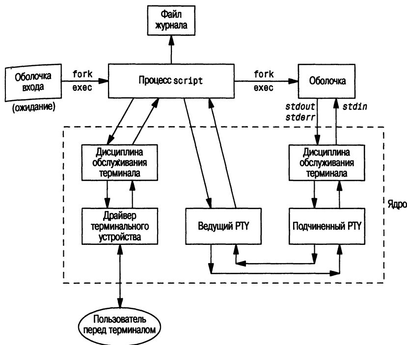
Рис. 19.4. Программа script
