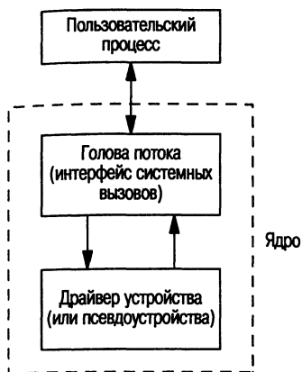
Рис. 14.4. Простейший поток
