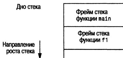
Рис. С.2. Раскладка фреймов стека при вызове функции vfork
