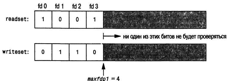
Рис. 14.9. Пример наборов дескрипторов для функции select
