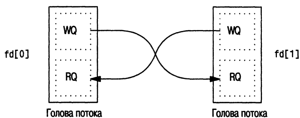
Рис. 17.2. Внутреннее устройство канала STREAMS
