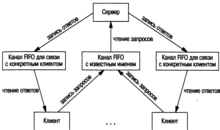
Рис. 15.12. Организация взаимодействий типа клиент-сервер с помощью каналов FIFO
