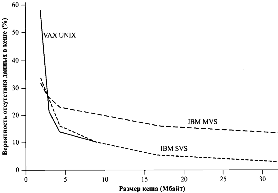
Рис. 11.10. Производительность дискового кеша при использовании LRU
