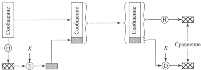
а) Использование симметричного шифрования
