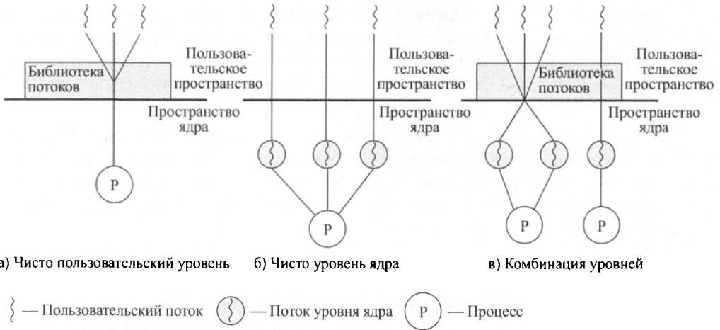
Рис. 4.5. Пользовательские потоки и потоки уровня ядра
