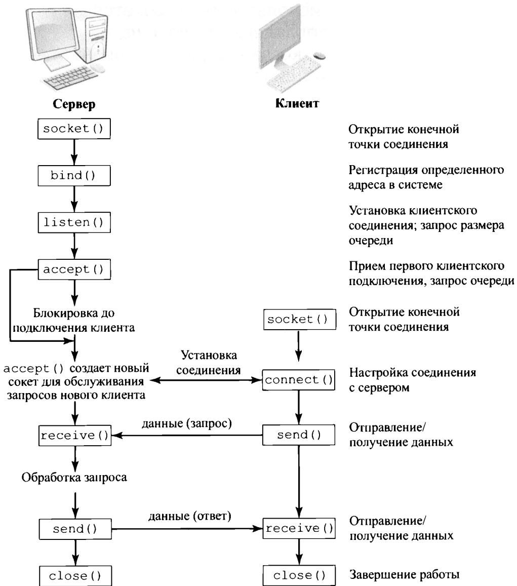
Рис. М.2. Системные вызовы сокетов для ориентированного на соединение протокола
