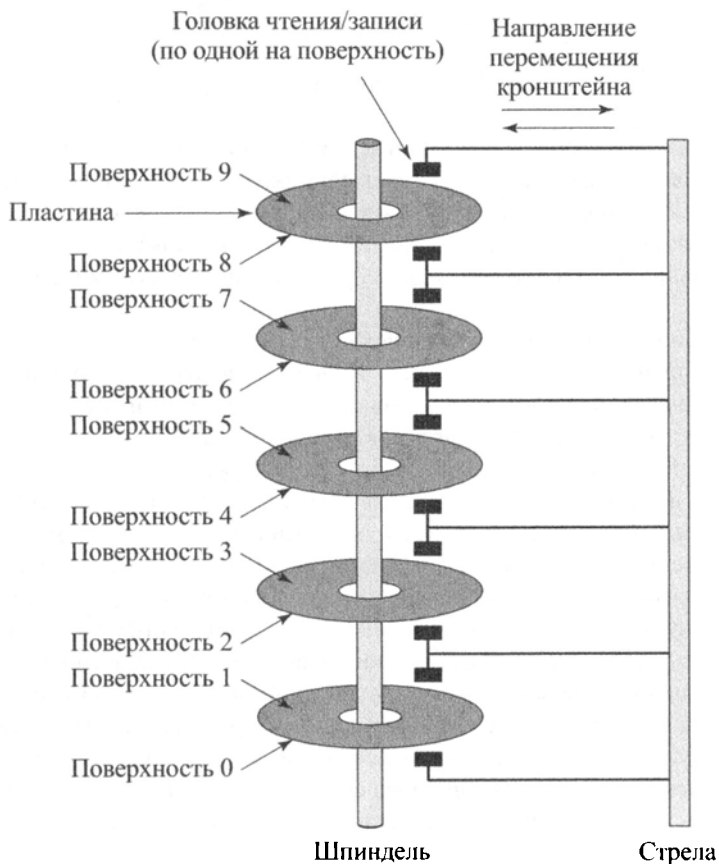
Рис. К.3. Компоненты магнитного диска
