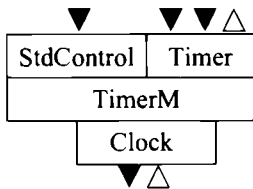
а) Компонент TimerM
