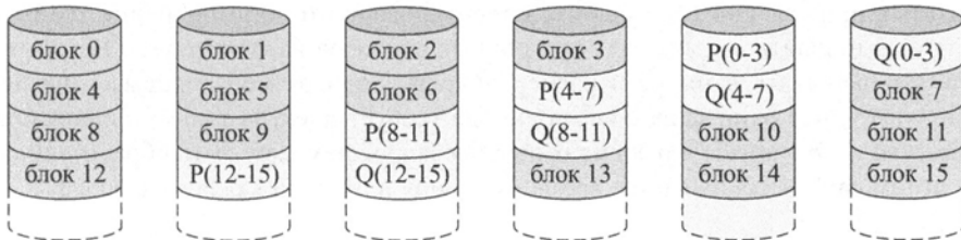
ж) RAID 6 (двойная распределенная четность с чередующимися блоками)
