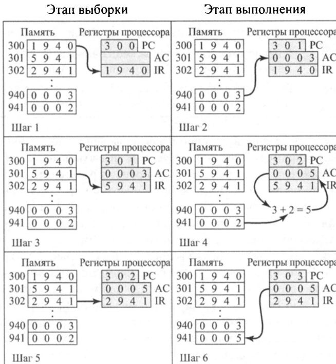
Рис. 1.4. Пример выполнения программы (содержимое памяти и регистров представлено шестнадцатеричными числами)
