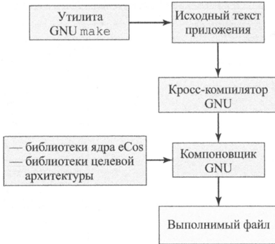
Рис. Р.3. Загрузка конфигурации eCos
