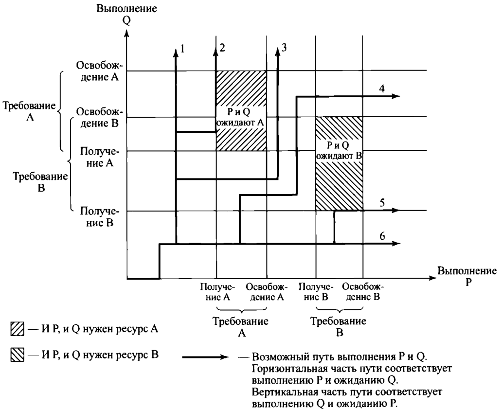
Рис. 6.3. Пример отсутствия взаимоблокировки [15]
