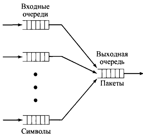
Рис. 21.10. Модель системы массового обслуживания для модуля сборки и разборки пакетов (PAD)
