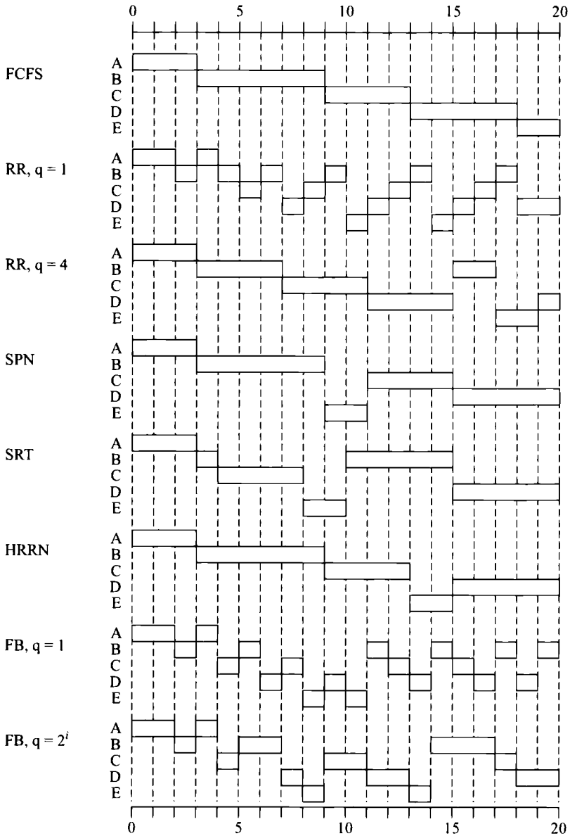
Рис. 9.5. Сравнение стратегий планирования
