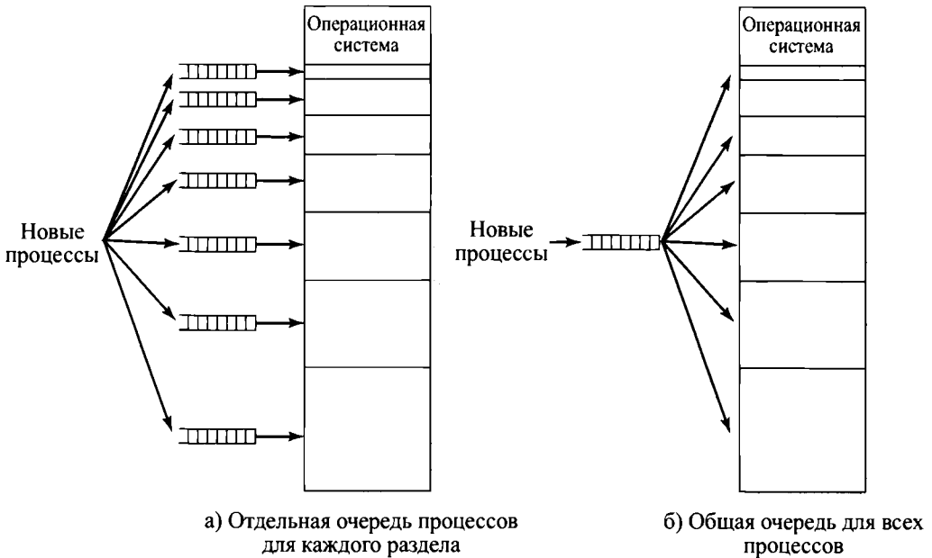
Рис. 7.3. Распределение памяти при фиксированном распределении
