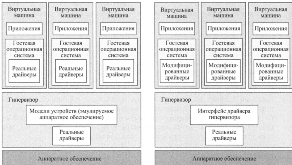
а) Гипервизор первого типа
