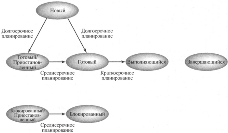
Рис. 9.1. Место планирования в диаграмме переходов состояний процесса
