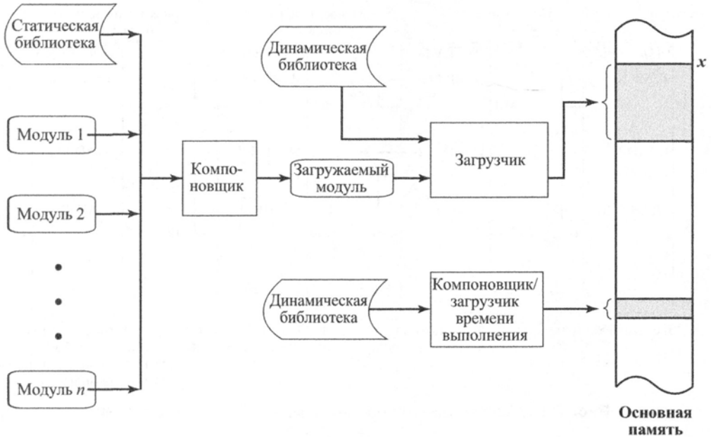
Рис. 7.14. Сценарий загрузки и связывания
