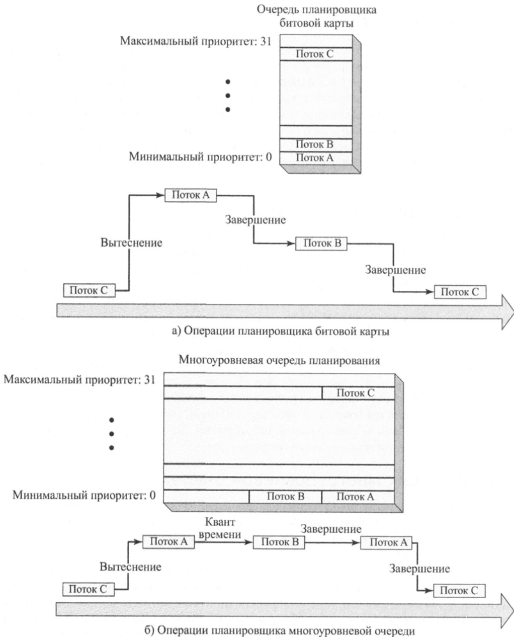
Рис. Р.6. Варианты планировщика eCos
