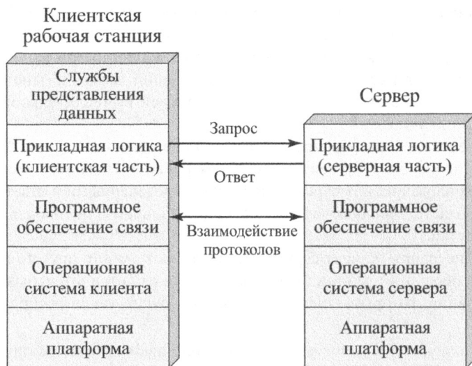
Рис. 18.2. Типичная архитектура "клиент/сервер"
