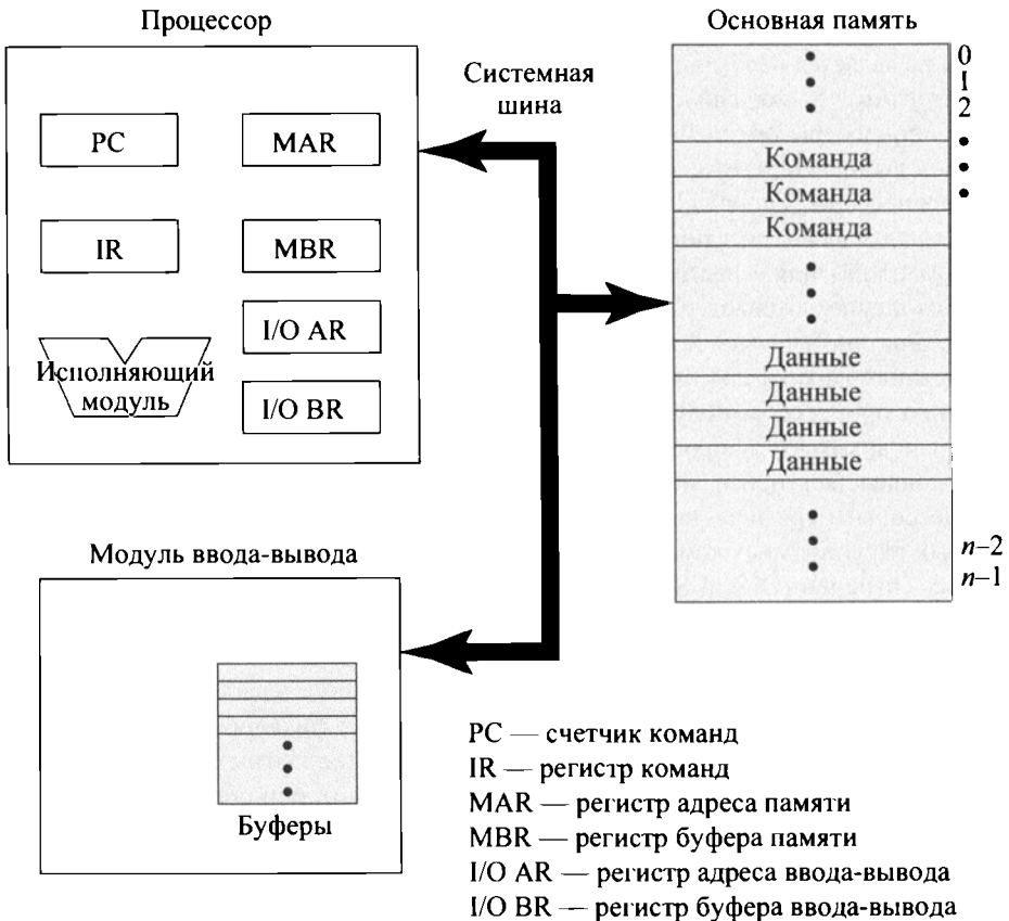
Рис. 1.1. Компоненты компьютера: общая структура
