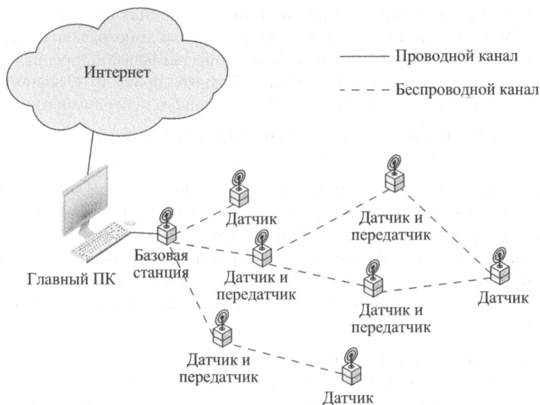
Рис. 13.8. Типичная топология сети беспроводных датчиков
