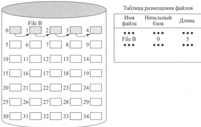
Рис. 12.12. Цепочечное размещение файлов (после уплотнения)
