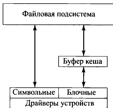
Рис. 11.12. Структура ввода-вывода в UNIX
