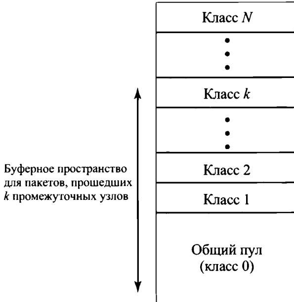
Рис. 19.18. Структурированный пул буферов для предотвращения взаимоблокировки
