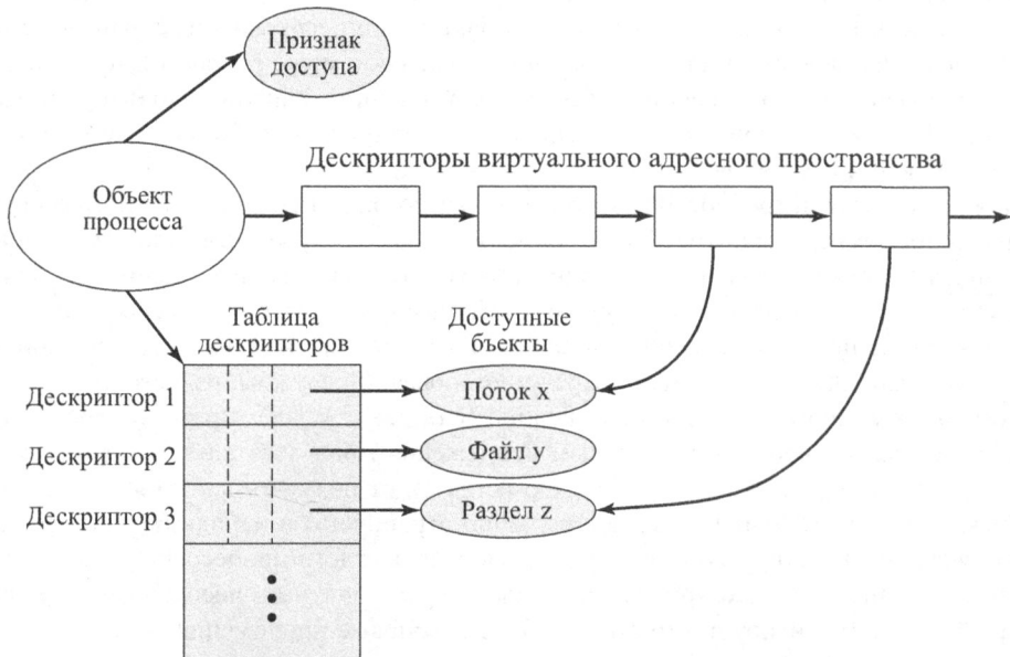
Рис. 4.10. Процессы Windows и их ресурсы
