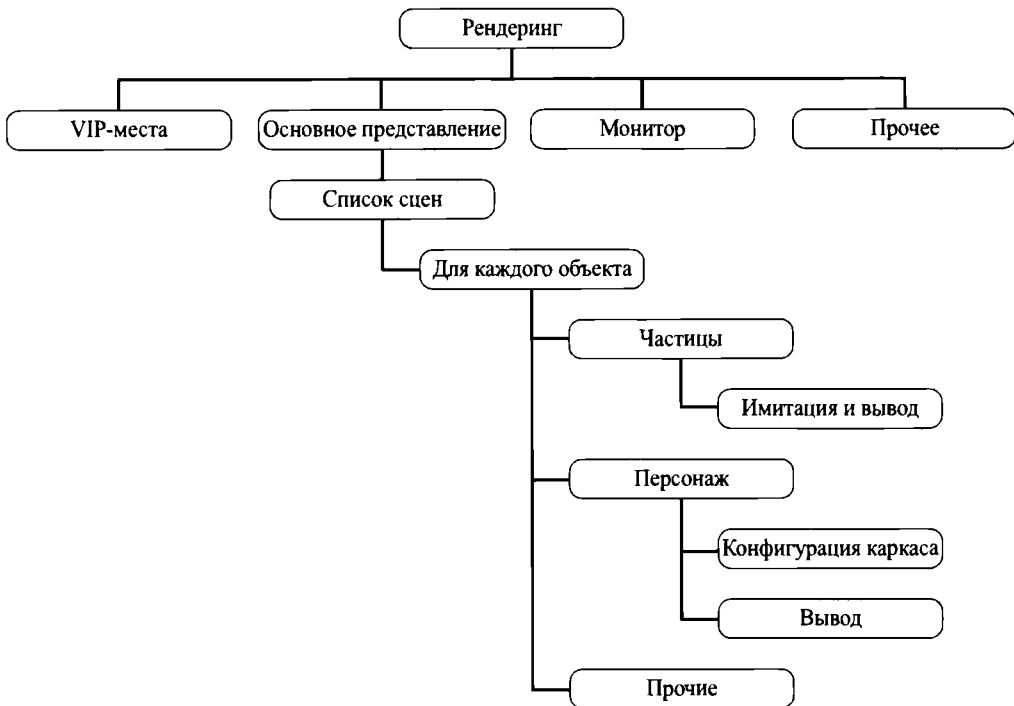
Рис. 4.9. Гибридная многопоточность для модуля рендеринга
