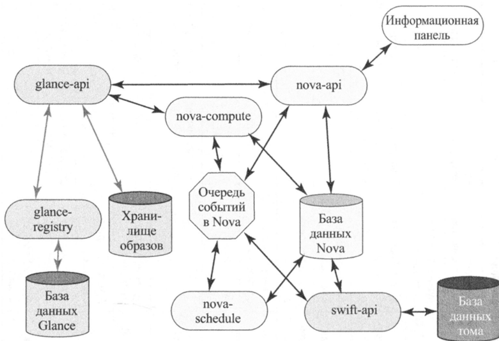
Рис. 16.10. Логическая архитектура компонента Nova
