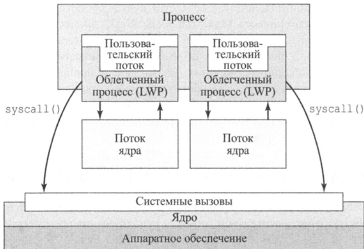
Рис. 4.12. Процессы и потоки в Solaris [167]
