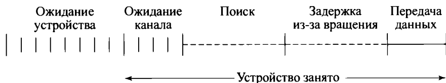
Рис. 11.6. Временная диаграмма работы диска
