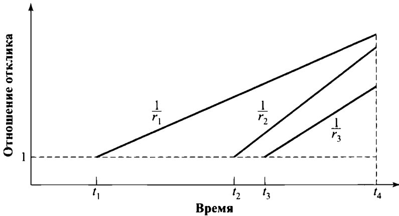
Рис. 9.18. Отношение отклика как функция времени
