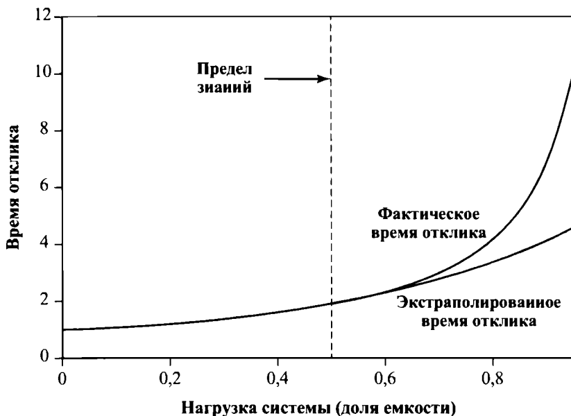
Рис. 21.1. Сравнение планируемого и фактического времени отклика
