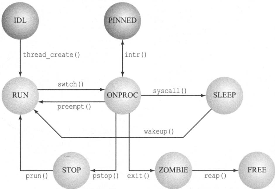
Рис. 4.14. Состояния потоков Solaris
