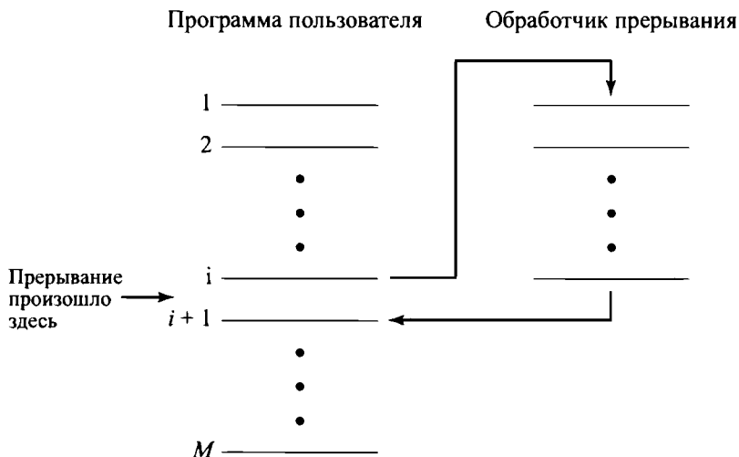
Рис. 1.6. Передача управления через прерывание
