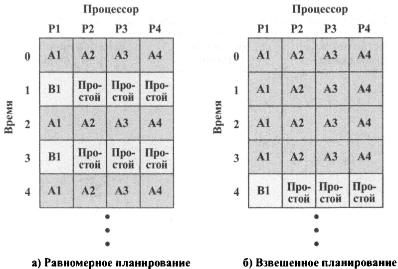
Рис. 10.2. Бригадное планирование
