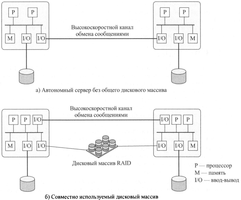
Рис. 18.13. Конфигурации кластеров
