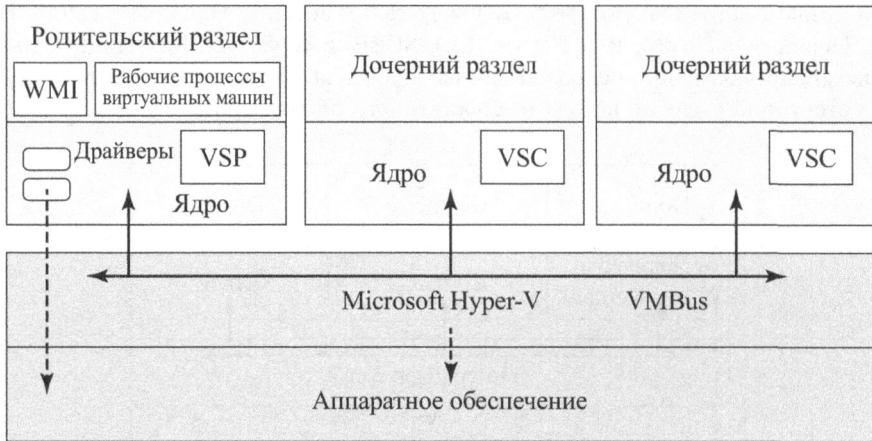
Рис. 14.11. Архитектура Hyper-V
