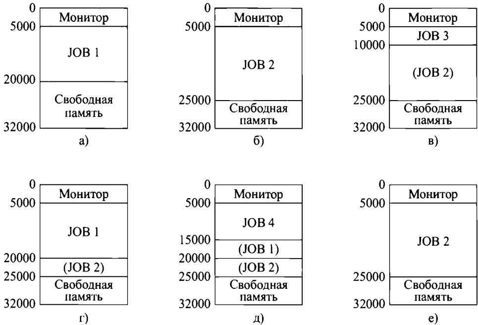
Рис. 2.7. Работа CTSS
