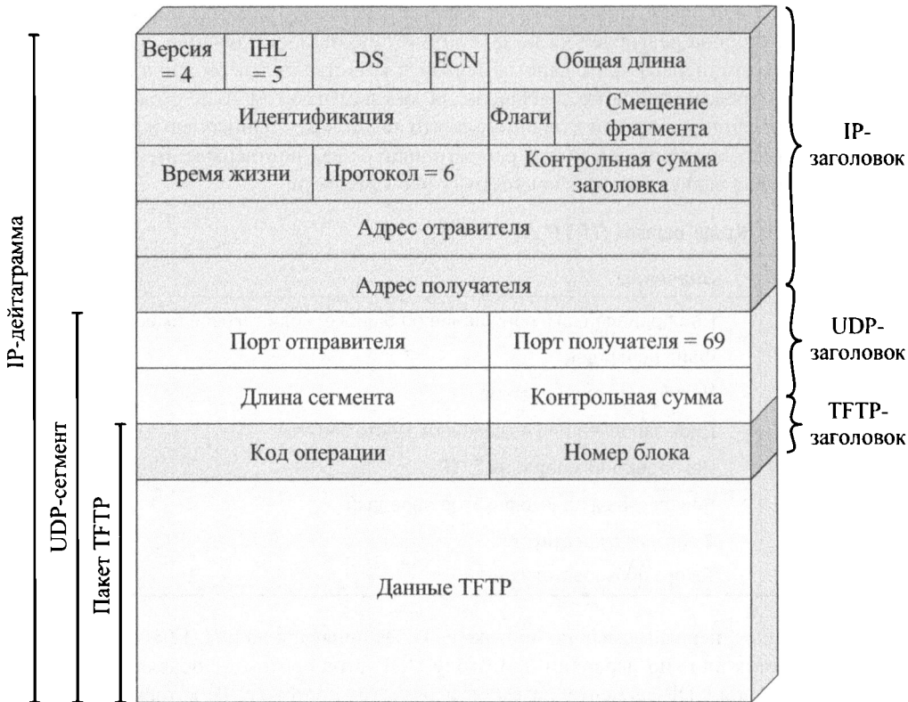
Рис. 17.10. Пакет TFTP
