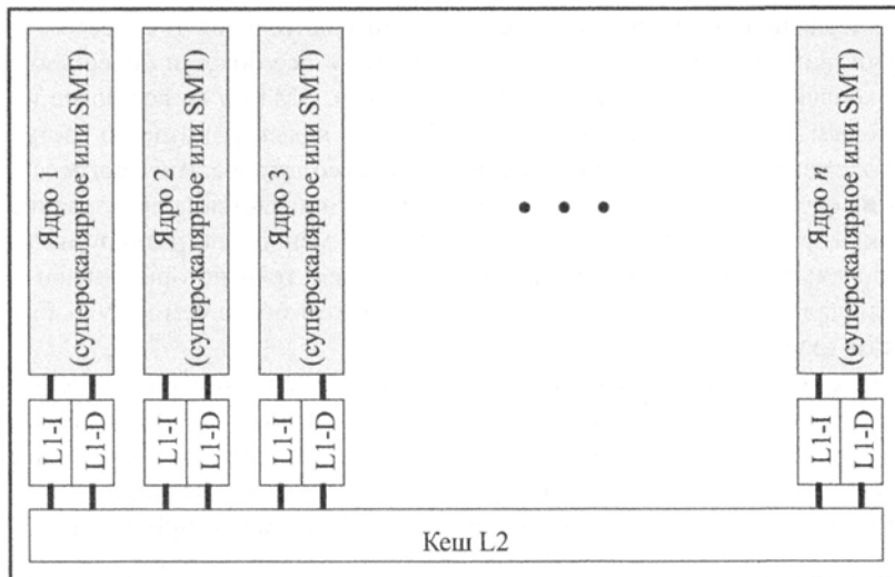
в) Многоядерность
