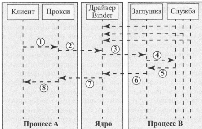
Рис. 6.16. Операции Binder
