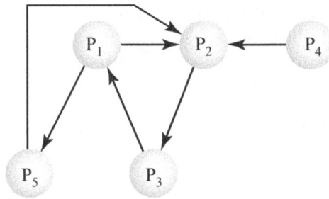
б) Взаимоблокировка
