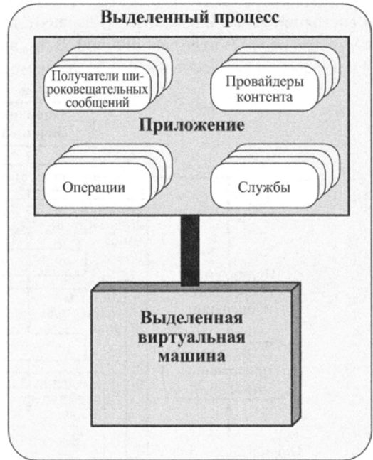
Рис. 4.16. Приложение Android
