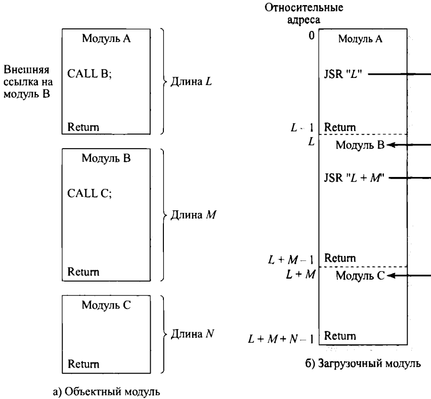
Рис. 7.16. Компоновка
