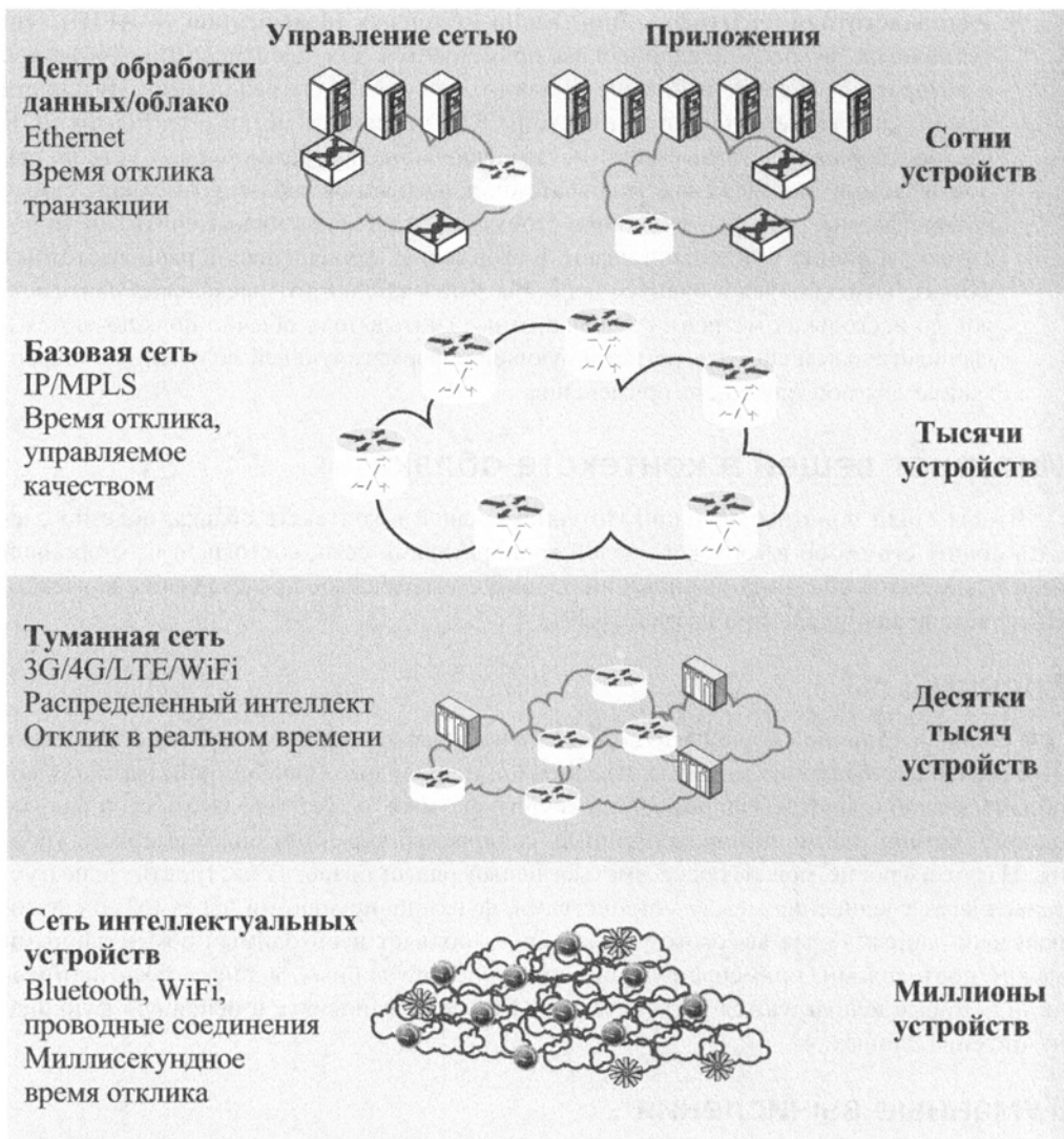
Рис. 16.12. Контекст Интернета вещей
