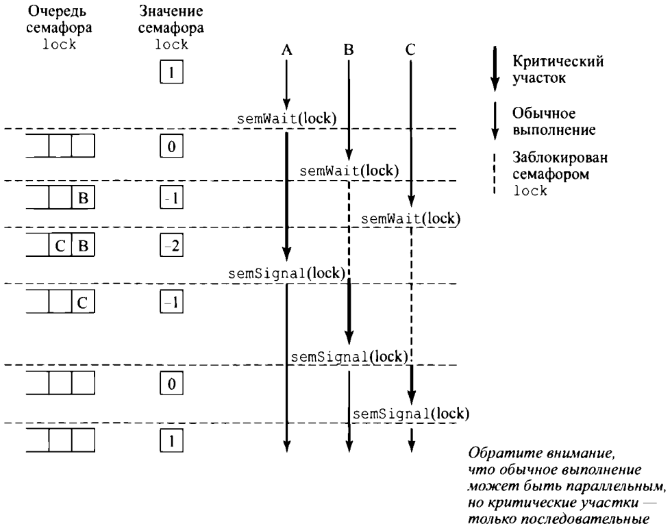
Рис. 5.10. Доступ процессов к общим данным, защищенным семафором
