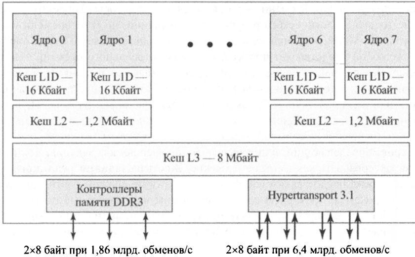
Рис. 10.3. Архитектура AMD Bulldozer
