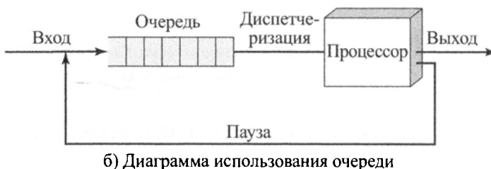
Рис. 3.5. Модель процесса с двумя состояниями
