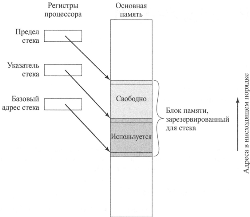
Рис. П.1. Типичная организация стека
