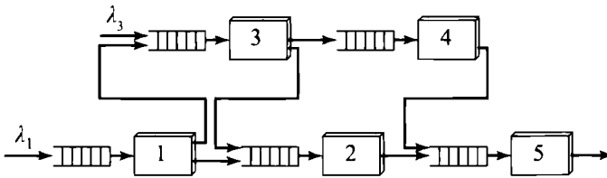
Рис. 21.7. Пример сети очередей
