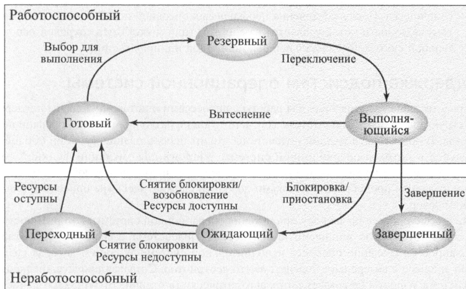
Рис. 4.11. Состояния потоков в операционной системе Windows
