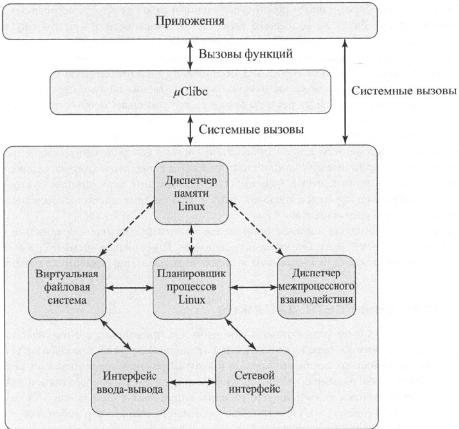
Рис. 13.7. Программная архитектура встроенной системы, построенной на основе \mu\text{Clinux} и \mu\text{Clibc}
