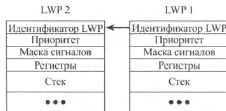
Рис. 4.13. Структура процесса в традиционном UNIX и в Solaris [154]
