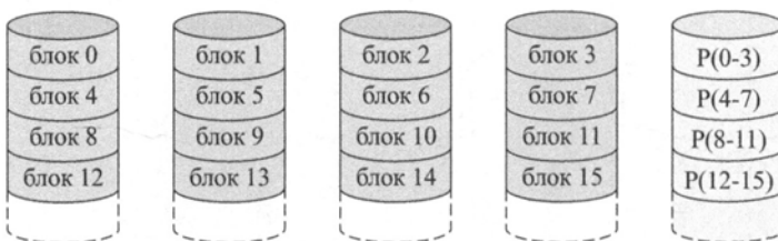
д) RAID 4 (четность с чередующимися блоками)
