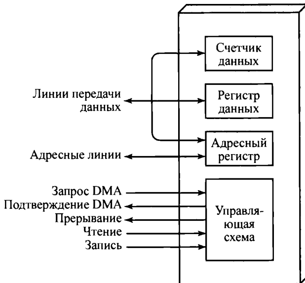
Рис. 11.2. Блок-схема прямого доступа к памяти
