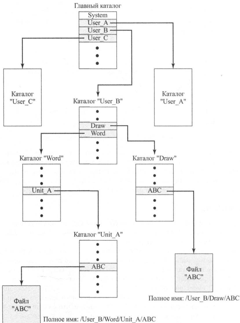
Рис. 12.7. Пример древовидной структуры каталога
