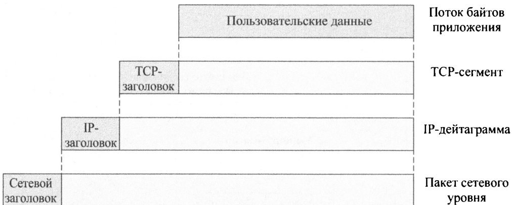
Рис. 17.5. Протокольные блоки данных (PDU) в архитектуре TCP/IP
