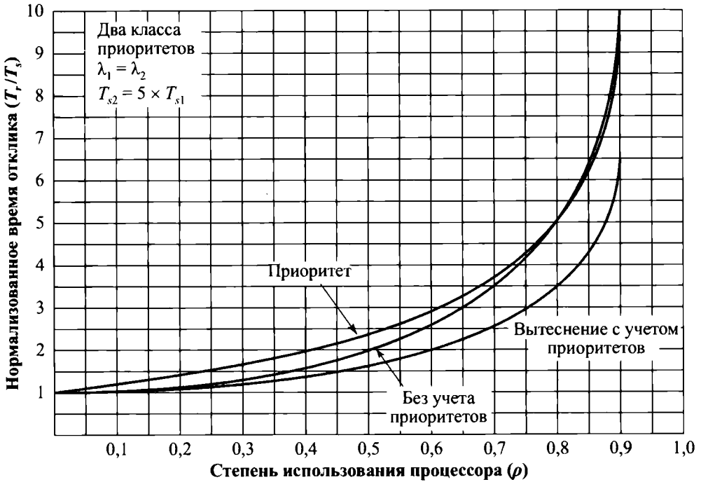
Рис. 9.11. Общее нормализованное время отклика
