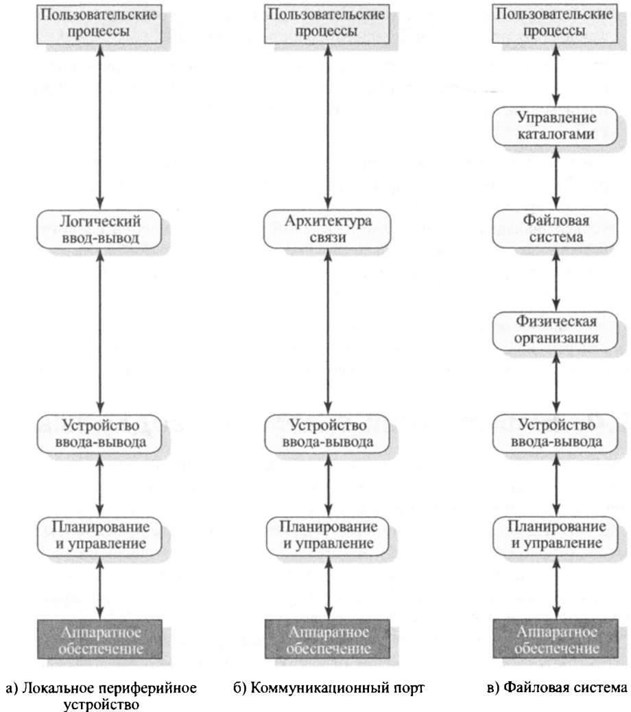
Рис. 11.4. Модель организации ввода-вывода
