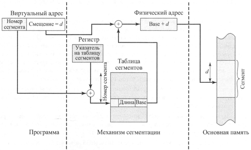
Рис. 8.11. Трансляция адреса в системе с сегментацией
