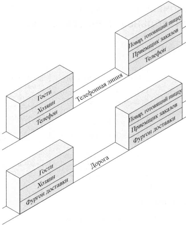
Рис. 17.8. Архитектура для задачи 17.1
