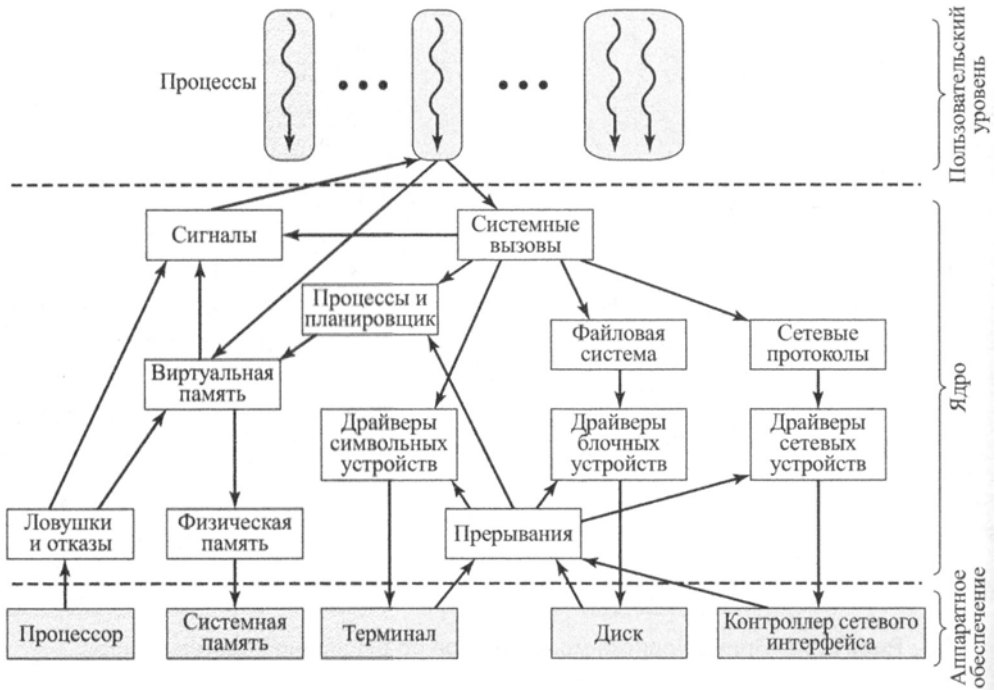
Рис. 2.19. Компоненты ядра Linux
