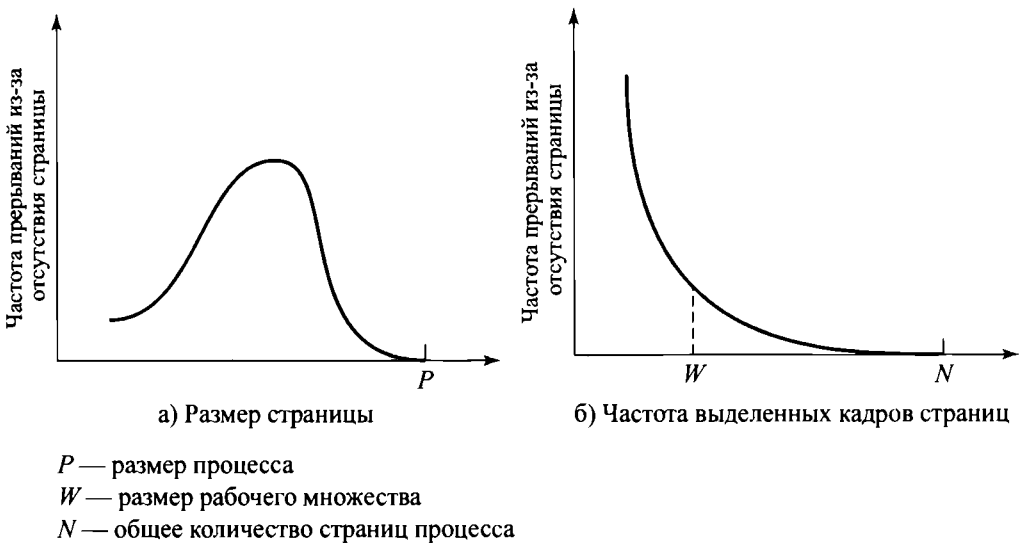
Рис. 8.10. Типичное поведение страничной организации
