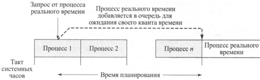
а) Круговое планирование с вытеснением
