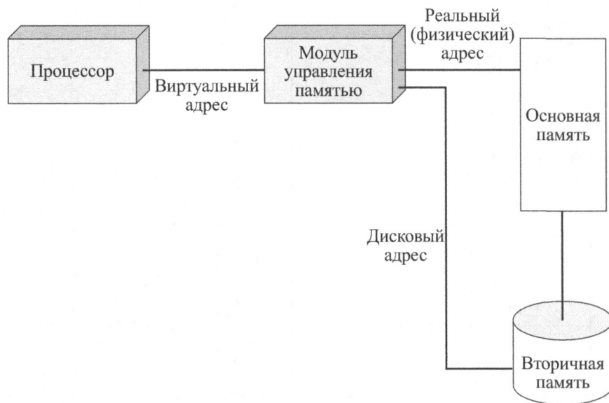
Рис. 2.10. Адресация виртуальной памяти
