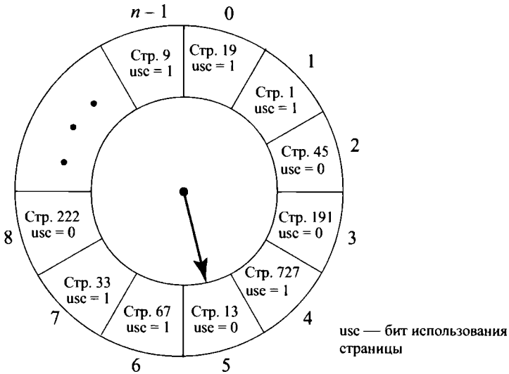
б) Состояние буфера непосредственно после замещения страницы
