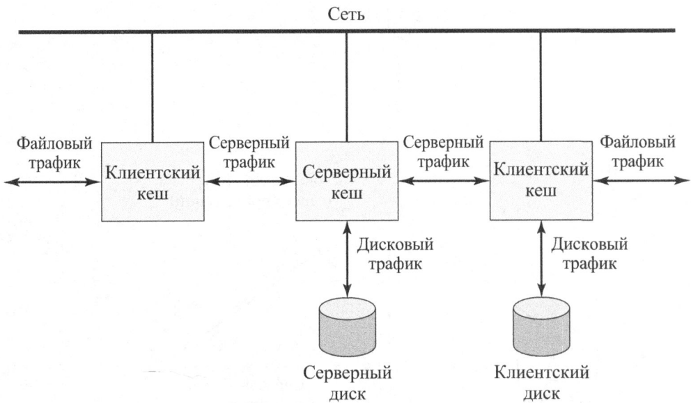
Рис. 18.7. Распределенное кеширование файлов в ОС Sprite
