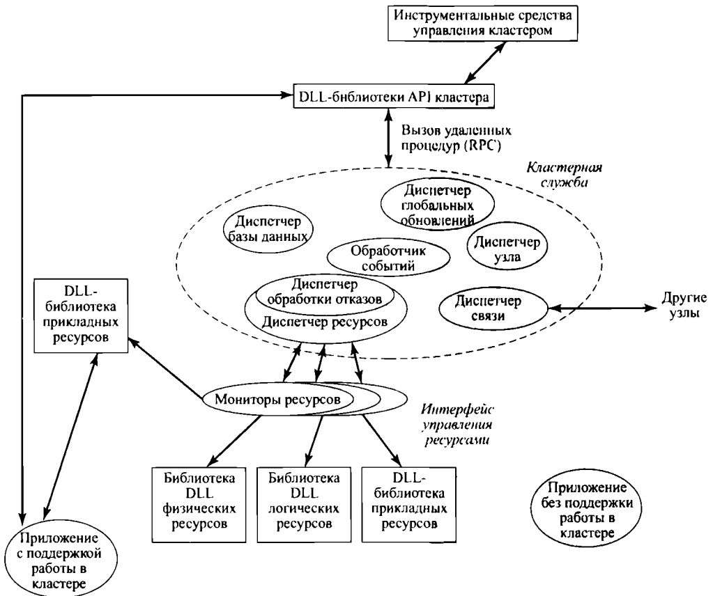
Рис. 18.15. Блок-схема кластерного сервера в Windows
