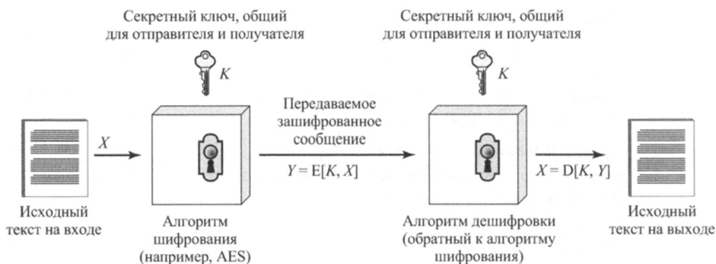
Рис. Л.1. Упрощенная модель симметричного шифрования
