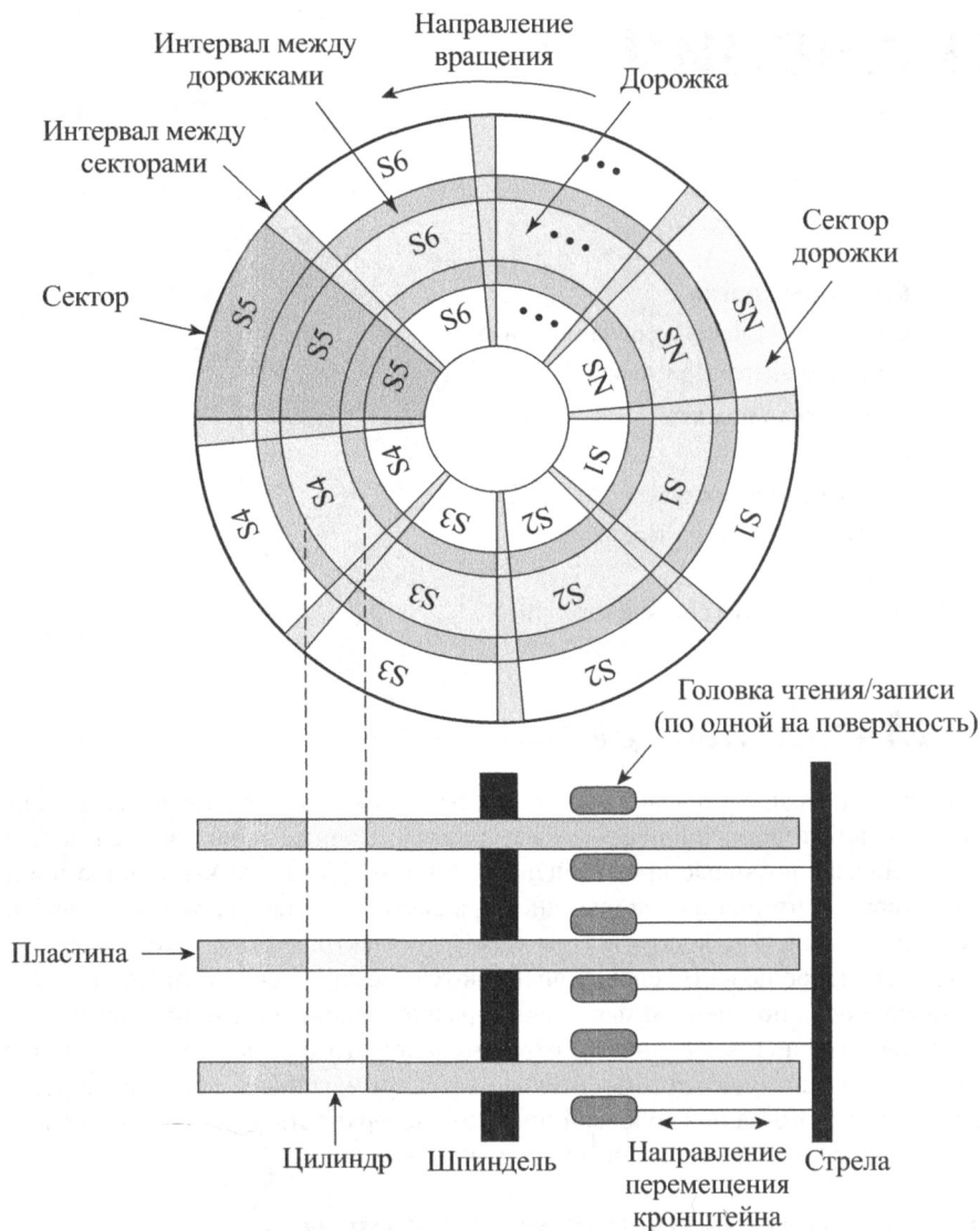
Рис. К.1. Схема размещения данных на диске
