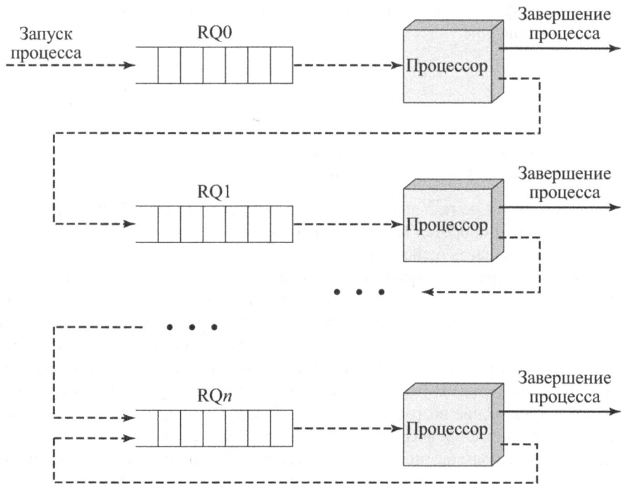
Рис. 9.10. Планирование со снижением приоритета
