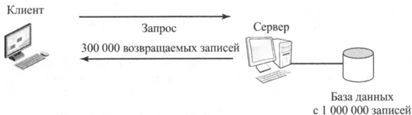
б) Неправильное применение архитектуры “клиент/сервер”
