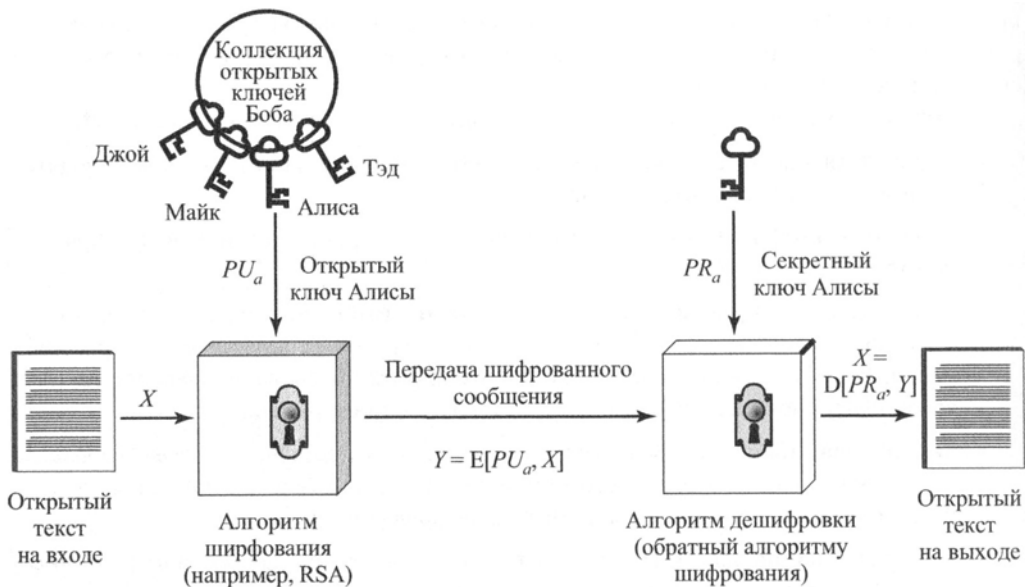
а) Шифрование с помощью открытого ключа
