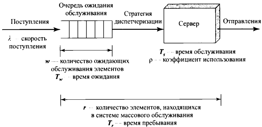
Рис. 21.2. Структура и параметры одноканальной системы массового обслуживания
