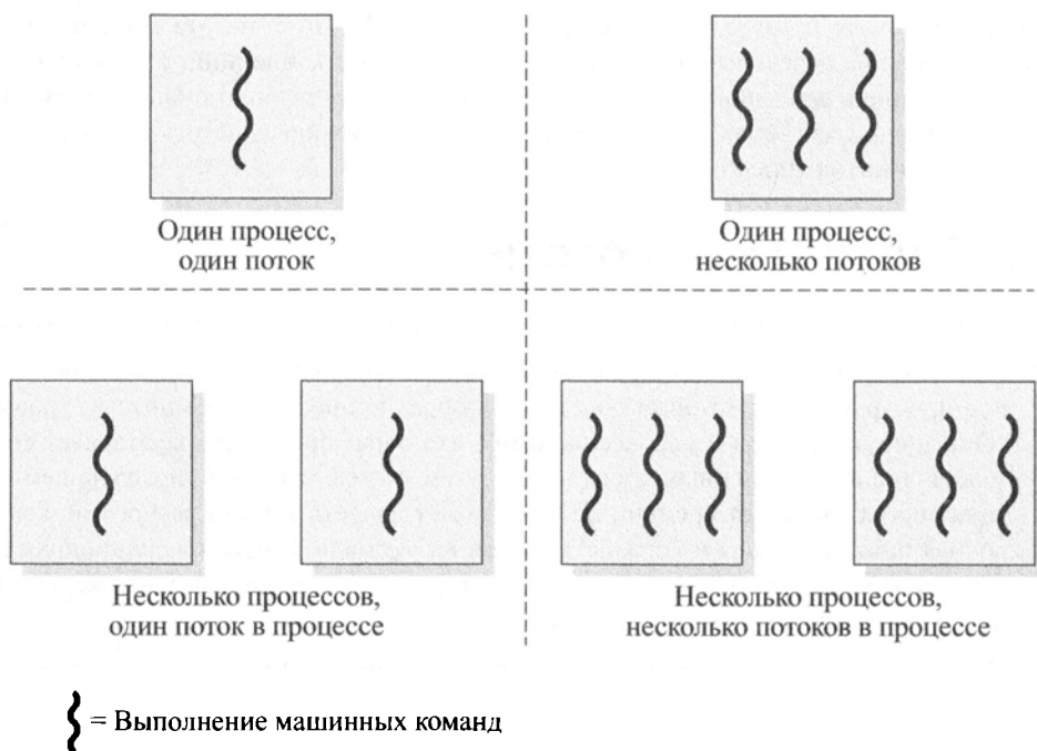
Рис. 4.1. Потоки и процессы
