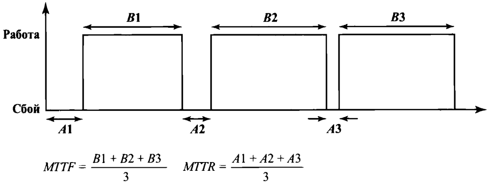
Рис. 2.13. Оперативное состояние системы
