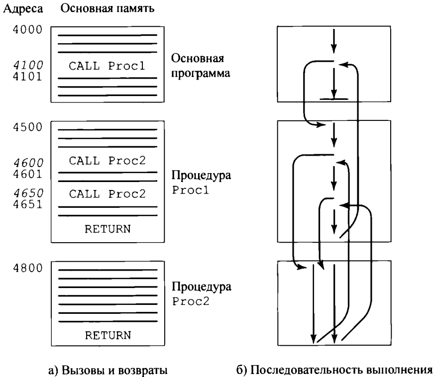
Рис. П.2. Вложенные вызовы процедур
