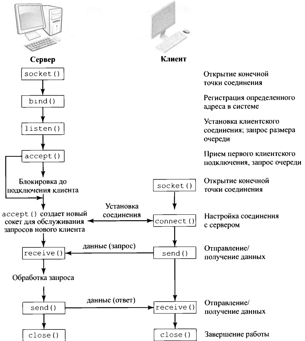
Рис. 17.6. Системные вызовы сокетов для ориентированного на соединения протокола
