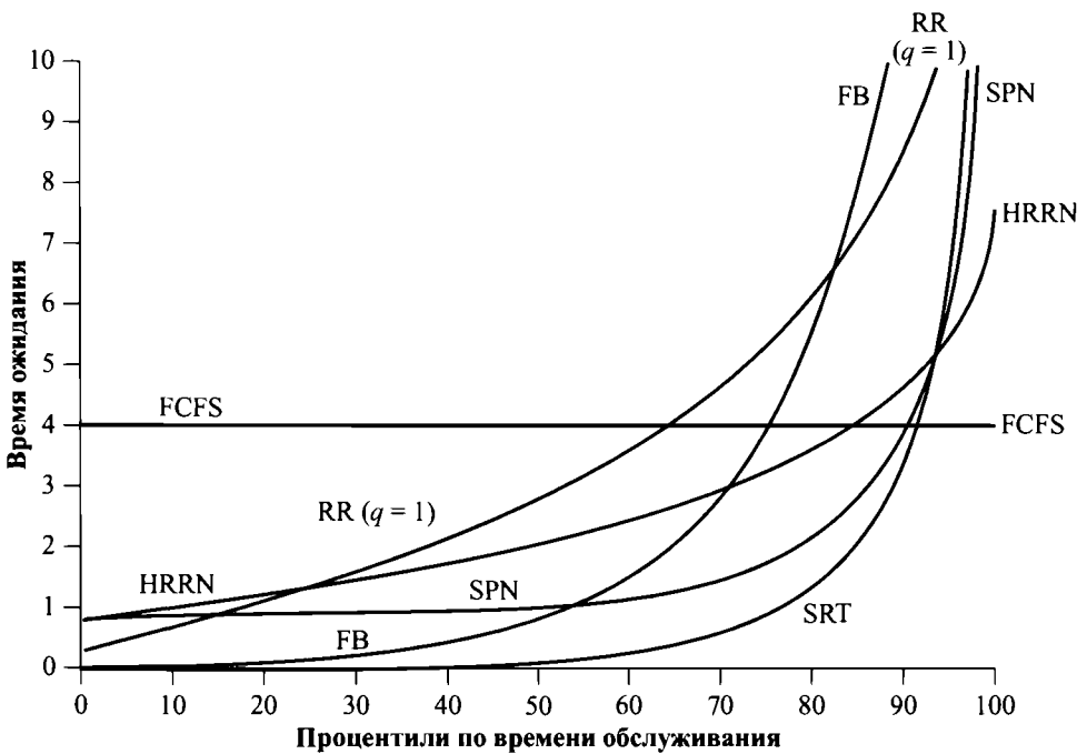
Рис. 9.15. Результаты имитационного моделирования для времени ожидания
