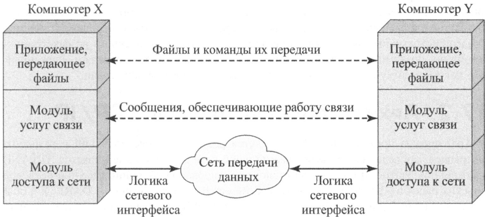
Рис. 17.1. Упрощенная архитектура для передачи файлов
