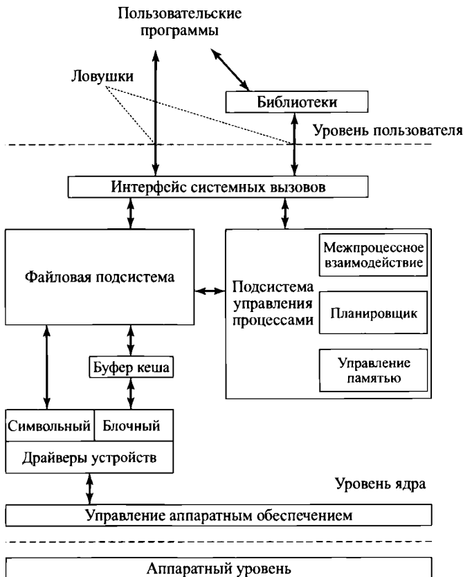
Рис. 2.15. Традиционная архитектура UNIX
