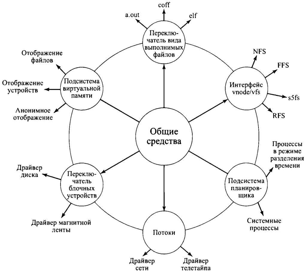
Рис. 2.16. Ядро современной системы UNIX
