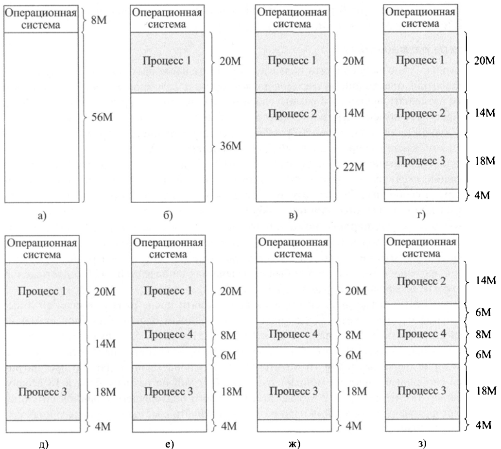
Рис. 7.4. Пример динамического распределения
