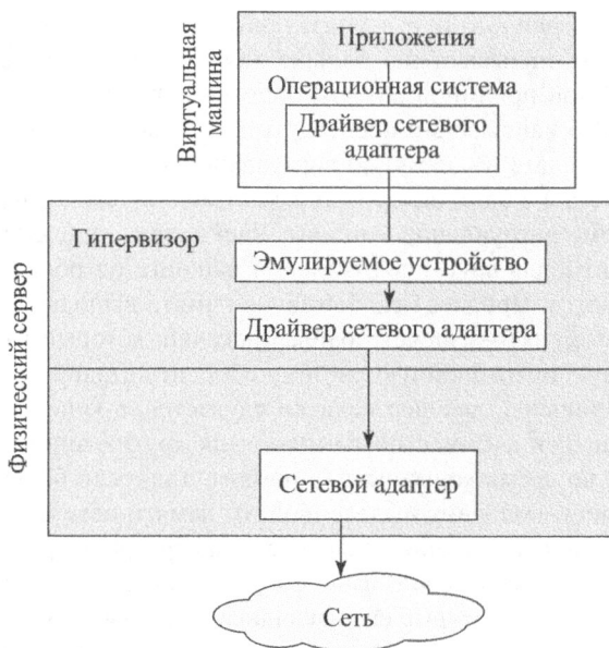
Рис. 14.8. Ввод-вывод в виртуальной среде
