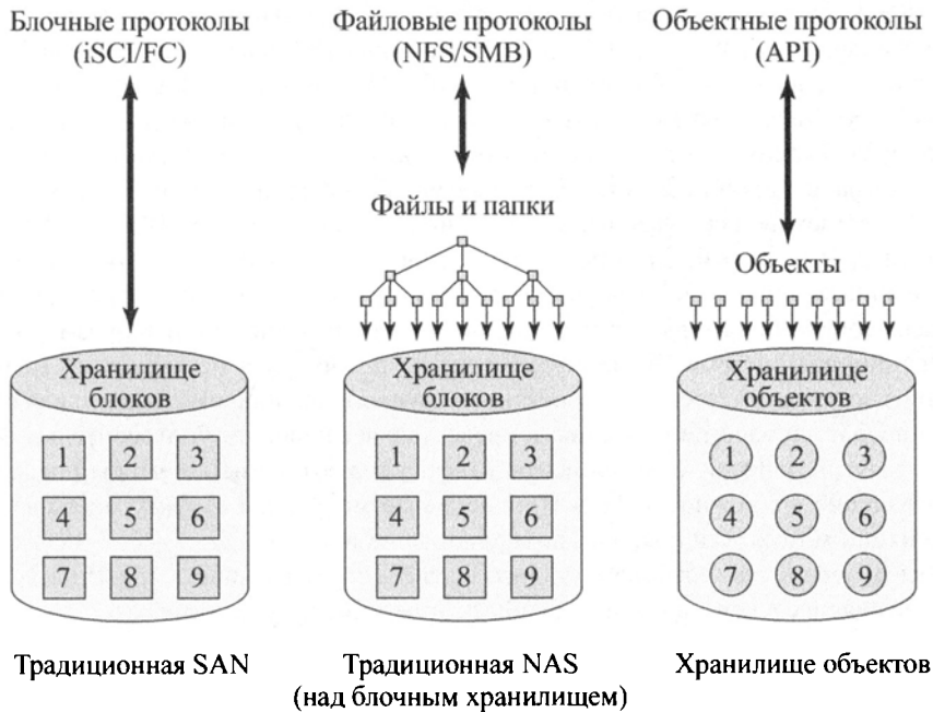
Рис. 16.8. Блочное, файловое и объектное хранение данных
