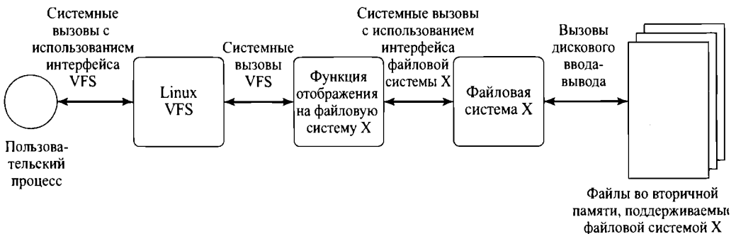
Рис. 12.18. Концепция VFS Linux
