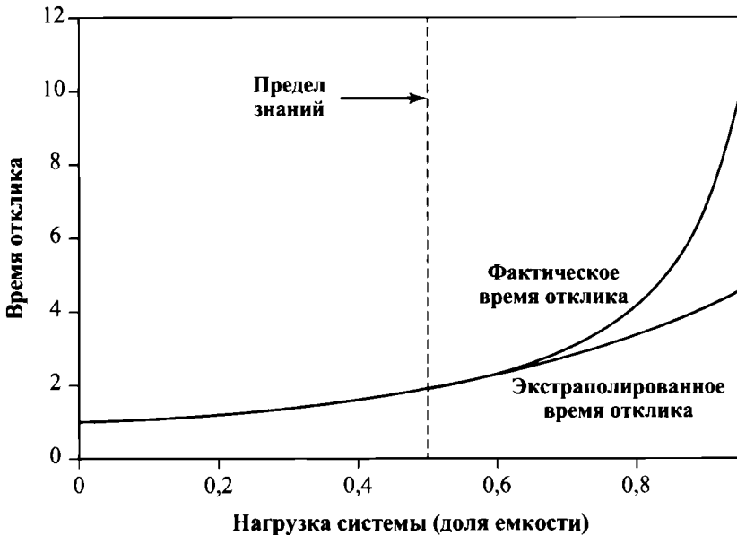
Рис. 3.1. Экстраполированное и фактическое время отклика
