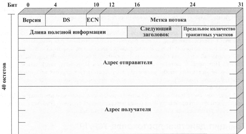
б) Заголовок пакета IPv6
