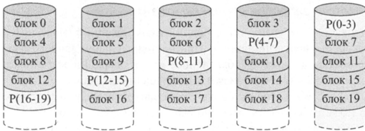
е) RAID 5 (распределенная четность с чередующимися блоками)
