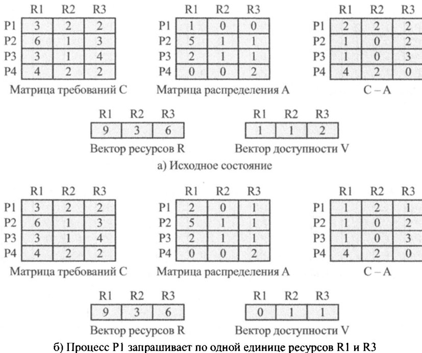
Рис. 6.8. Определение опасного состояния
