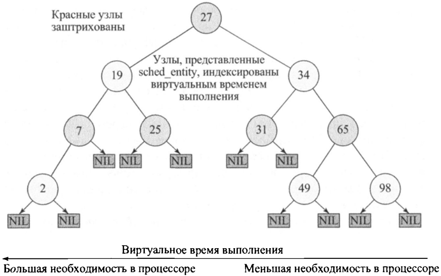
Рис. 10.11. Пример применения красно-черного дерева для CFS
