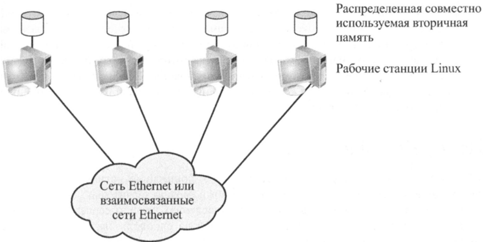
Рис. 18.16. Типичная конфигурация Beowulf
