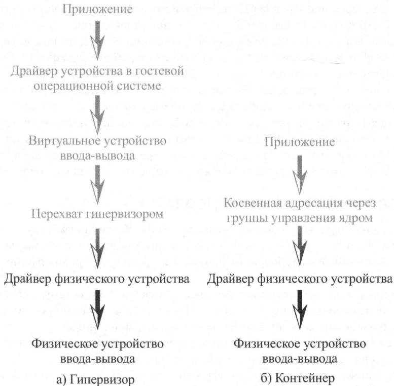
Рис. 14.5. Прохождение потока данных в операции ввода-вывода через гипервизор и контейнер
