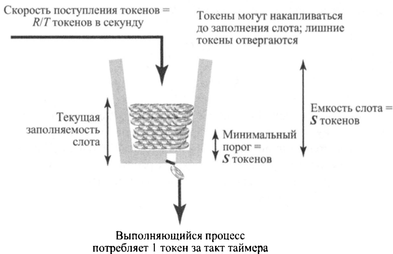
Рис. 14.13. Схематическое представление маркерного слота в Linux VServer
