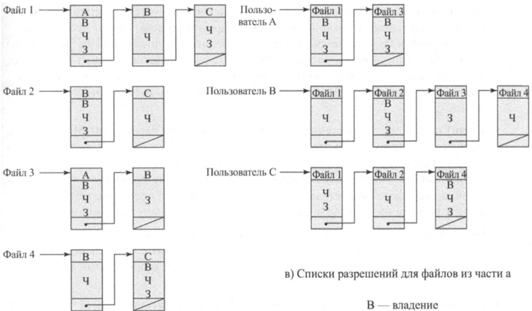
б) Списки управления доступом к файлам из части а
