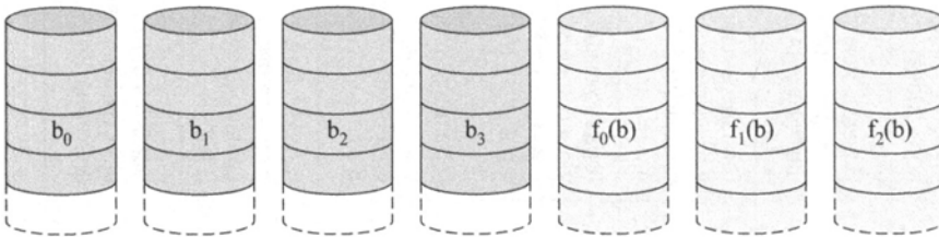
в) RAID 2 (избыточность с кодами Хэмминга)
