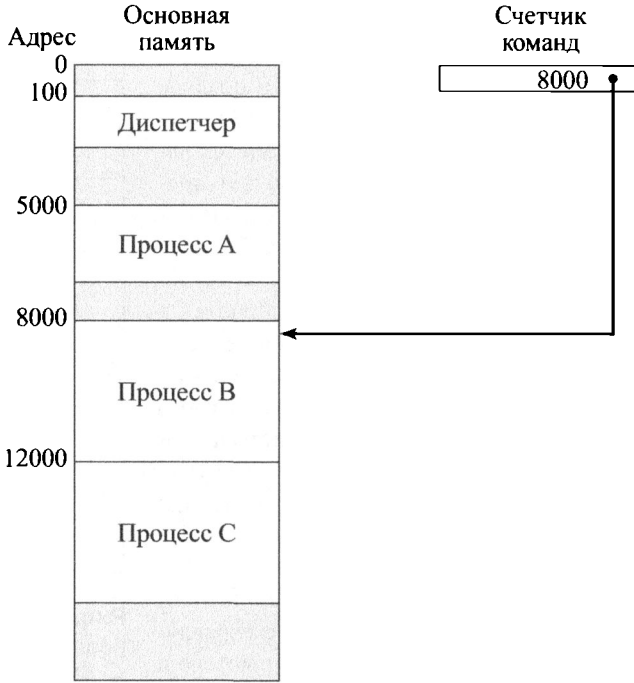
Рис. 3.2. Состояние системы в момент выполнения 13-го командного цикла
