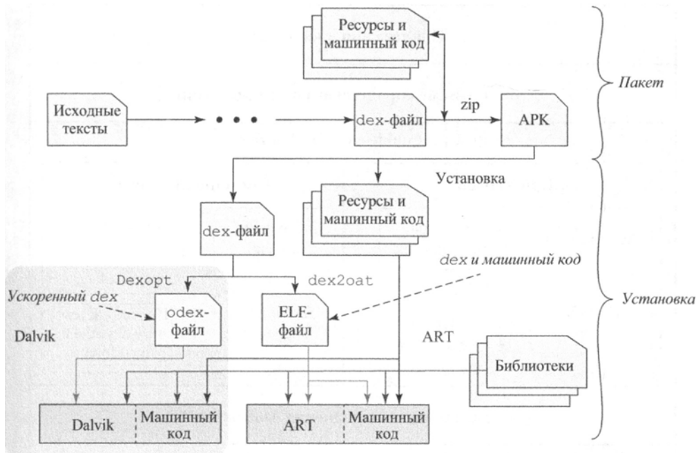
Рис. 2.21. Жизненный цикл APK
