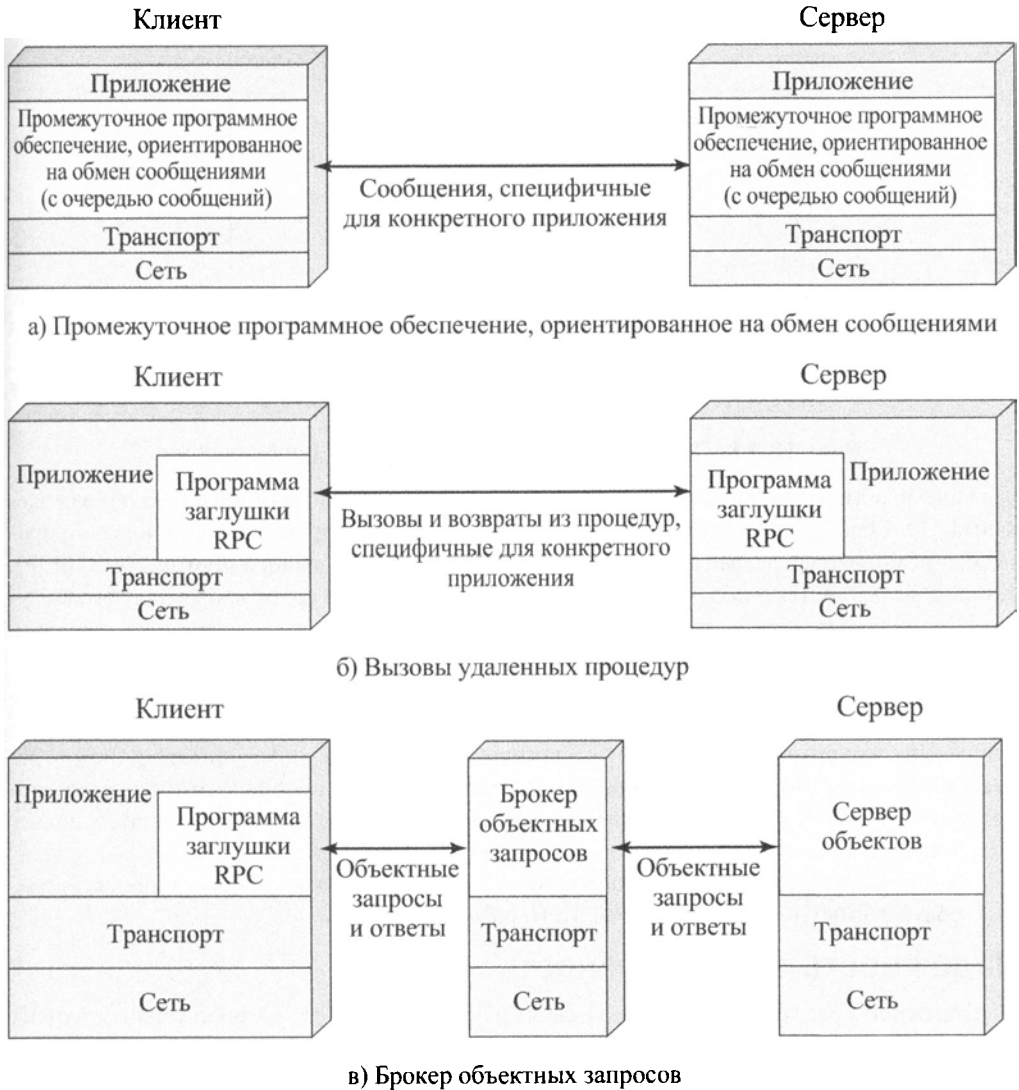
Рис. 18.10. Механизмы ППО для обмена сообщениями
