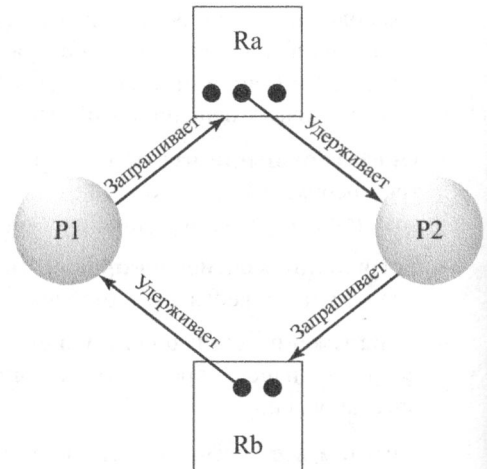
г) Отсутствие взаимоблокировки
