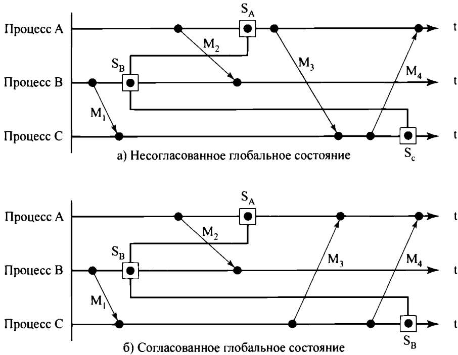
Рис. 19.4. Несогласованные и согласованные глобальные состояния
