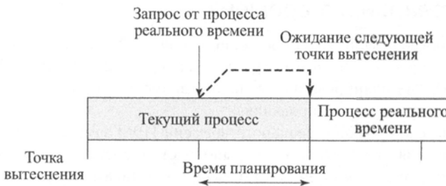
в) Вытесняющее планирование на основе приоритетов с точками вытеснения
