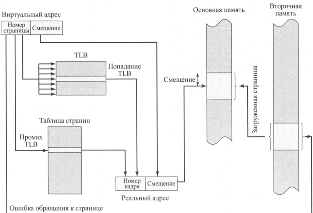
Рис. 8.6. Использование TLB
