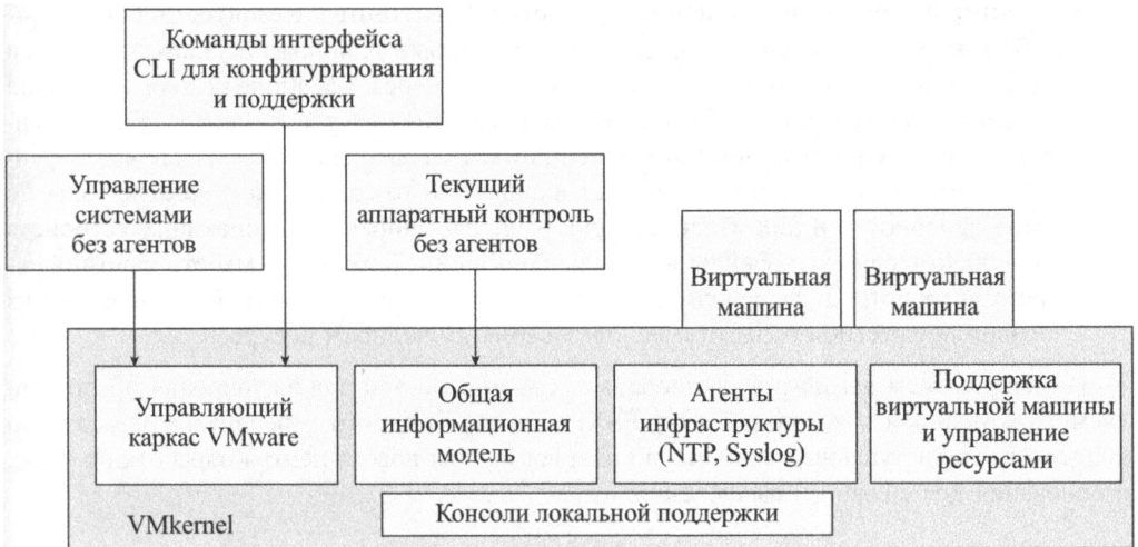
б) ESXi
