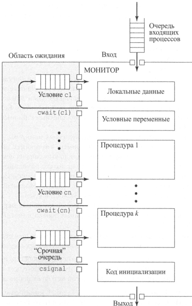
Рис. 5.18. Структура монитора
