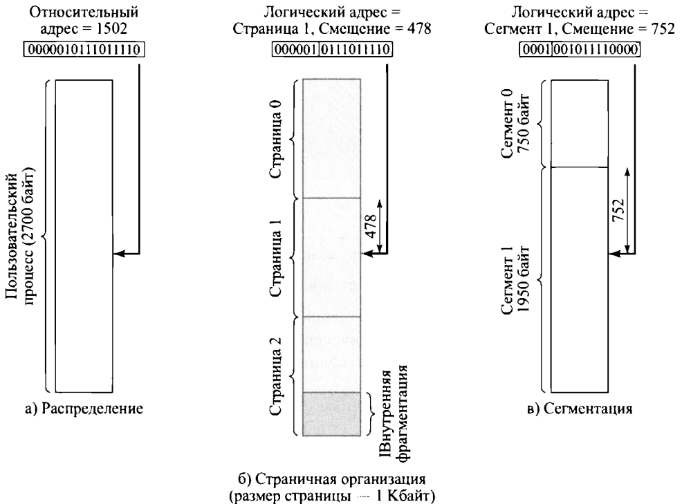
Рис. 7.11. Логические адреса
