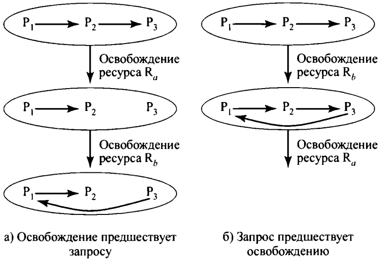
Рис. 19.12. Фантомная блокировка
