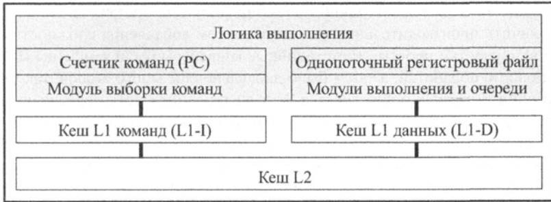
а) Суперскалярность
