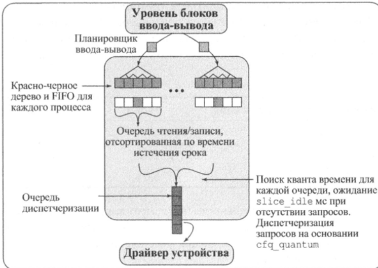
Планировщик CFQ
