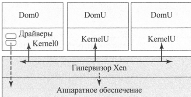
Рис. 14.10. Архитектура Xen
