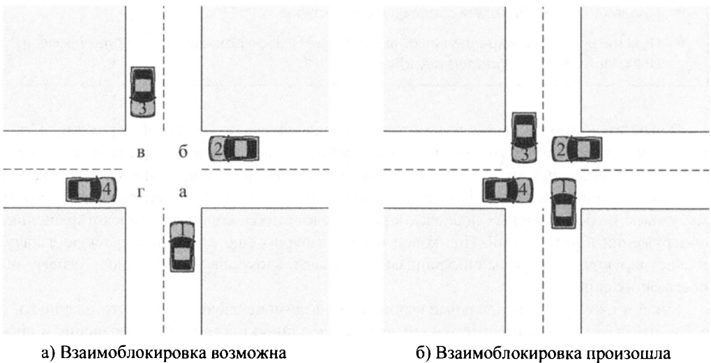
Рис. 6.1. Пример взаимоблокировки
