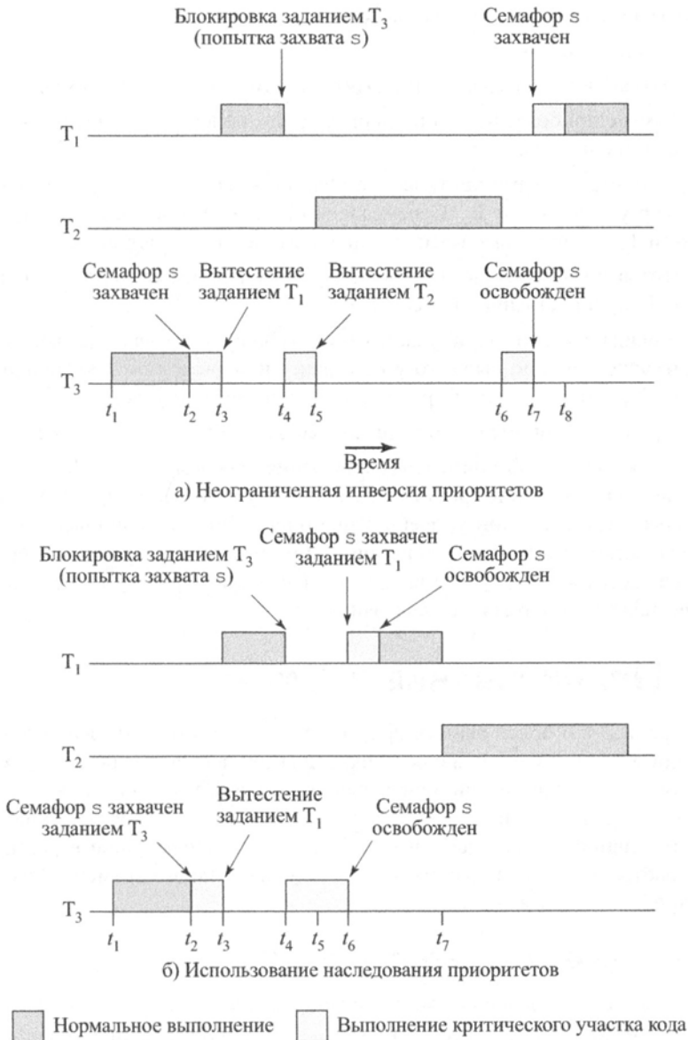
Рис. 10.9. Инверсия приоритетов
