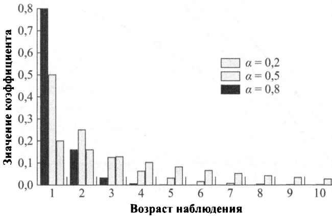
Рис. 9.8. Весовые коэффициенты при разных значениях \alpha
