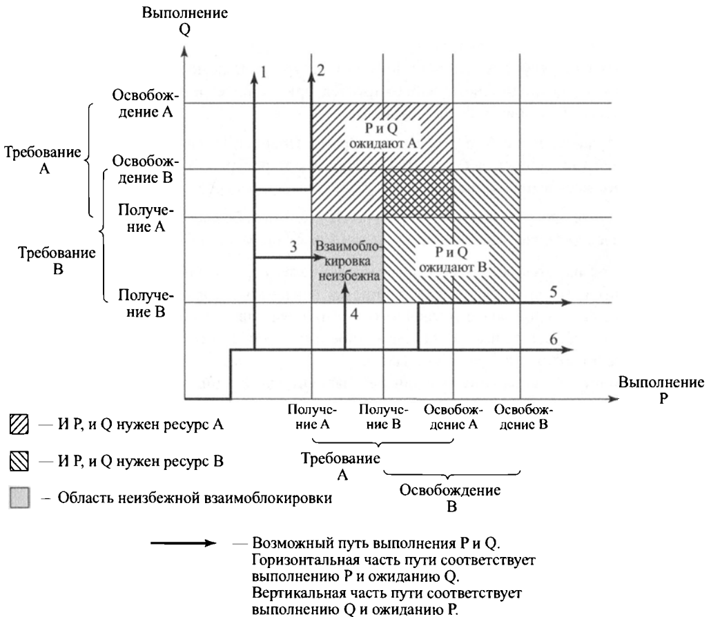
Рис. 6.2. Пример взаимоблокировки
