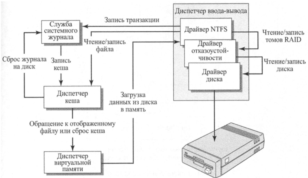
Рис. 12.20. Компоненты NTFS
