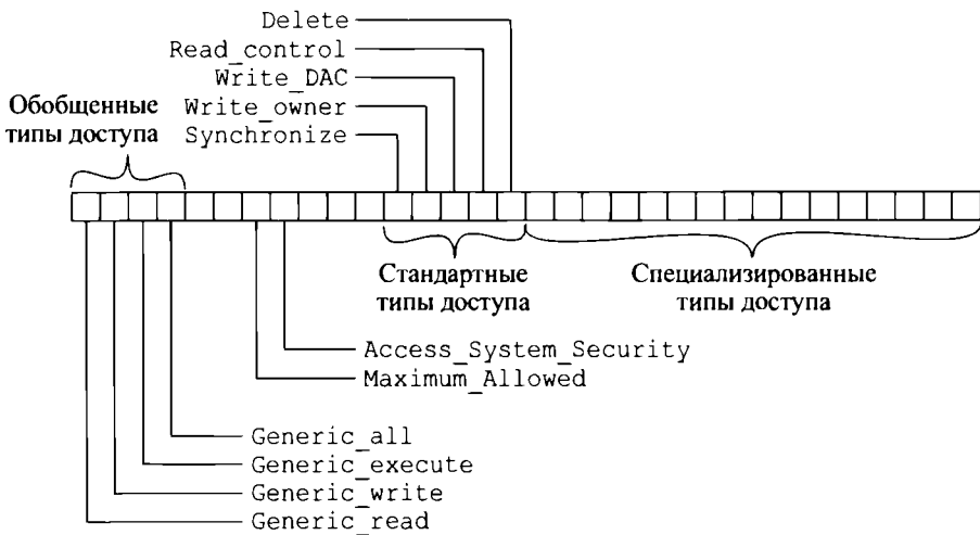
Рис. 15.10. Маски доступа
