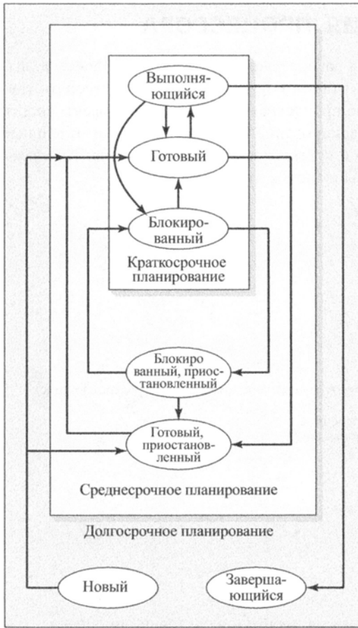
Рис. 9.2. Уровни планирования
