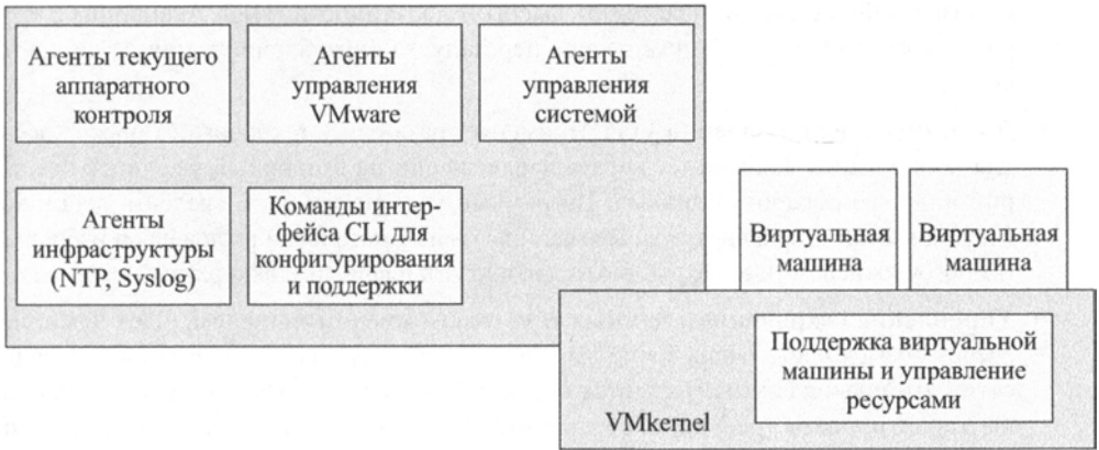
а) ESX
