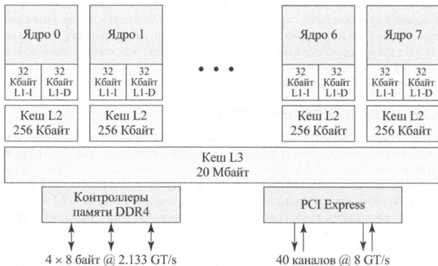
а) Блок-схема
