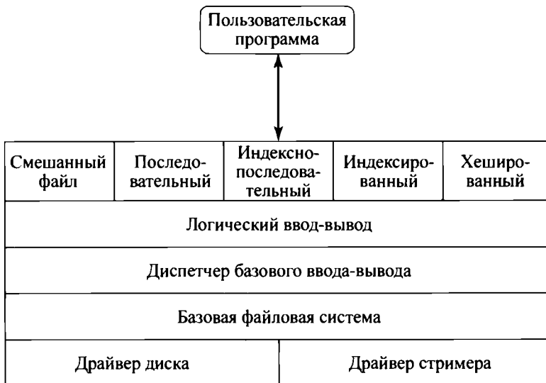
Рис. 12.1. Архитектура программного обеспечения файловой системы [95]
