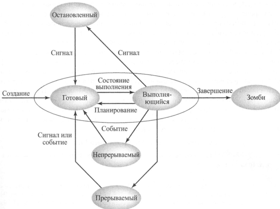
Рис. 4.15. Модель процессов и потоков Linux
