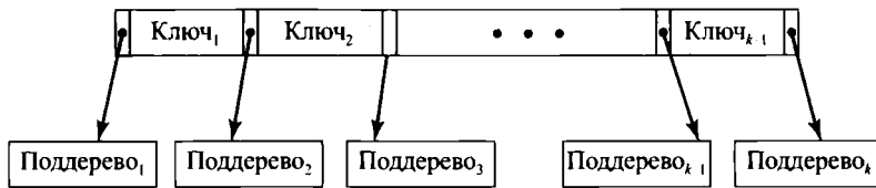
Рис. 12.4. Узел В-дерева с k дочерними узлами
