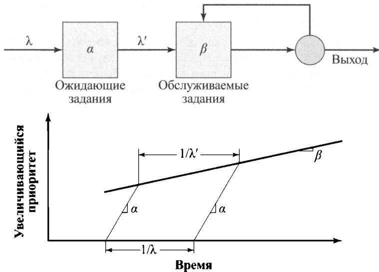
Рис. 9.19. Эгоистичное круговое планирование
