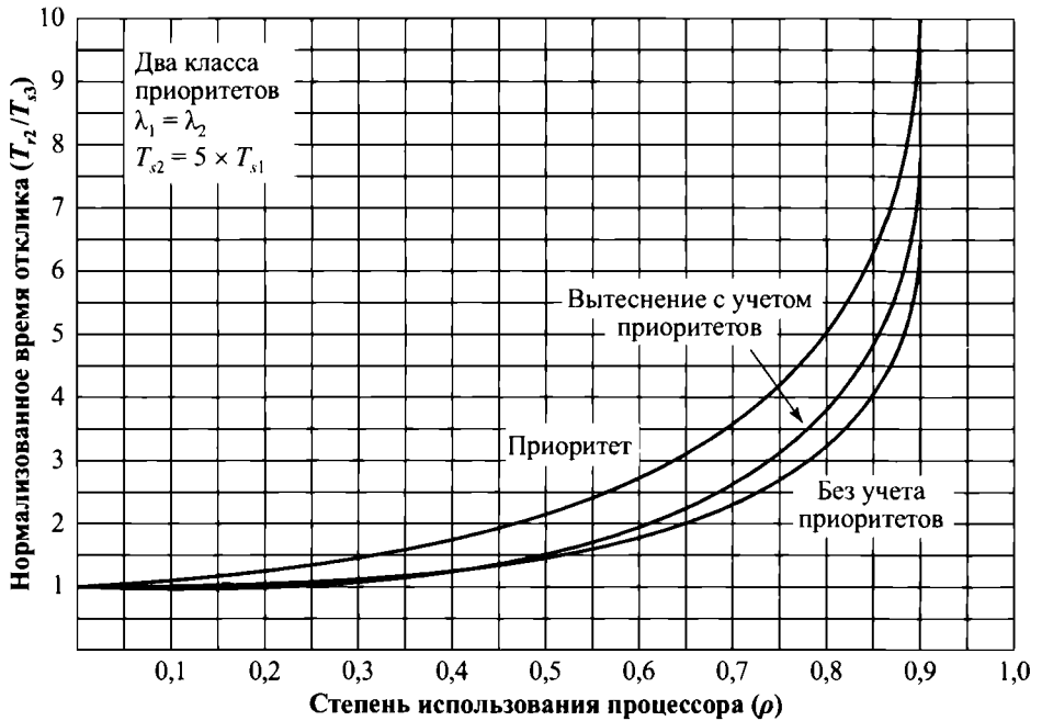
Рис. 9.13. Нормализованное время отклика для длинных процессов
